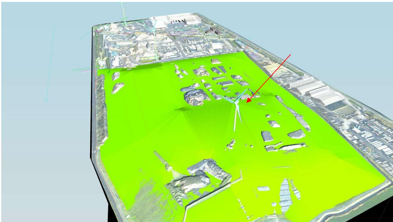
Figuur 2-2: Vogelvlucht weergave van het Sortiva-terrein vanuit het zuiden met daarop de voorgenomen locatie van de derde windturbine gevisualiseerd [REF5]
