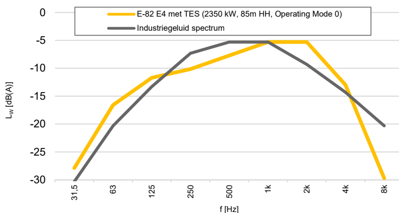
figuur 3 vergelijking spectra windturbines met een voorbeeld industriespectrum 4
