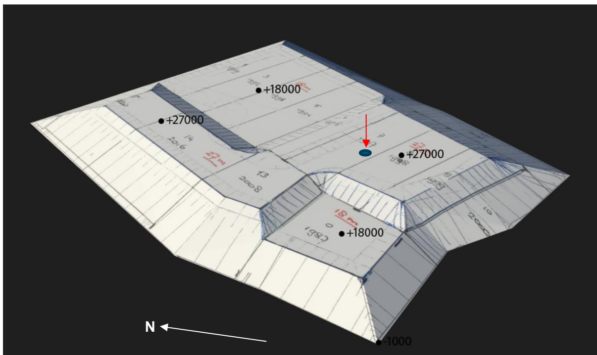
Figuur 3-1: maatvoering deponie (bron Sortiva, bestand 'Deponie na 2030 met stortvakken nieuwe versie 2013.png')
