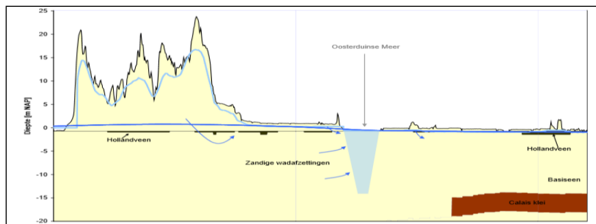
Figuur 11: Een doorsnede van het Oosterduinse kanaal met zijn omgeving. Zichtbaar zijn de Hollandveen lagen en, met blauwe peilen aangegeven, de lokale grondwater stroom richting
