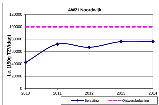
Figuur 5 – gemeten biologische belasting AWZI Noordwijk
