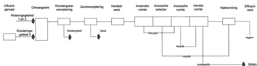
Afbeelding 1: Proces Flow Diagram (PFD) van waterlijn AWZI Noordwijk. In totaal zijn er twee identieke straten aanwezig (vanaf anaerobe ruimte tot en met nabezinktank)
