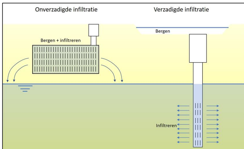
Figuur 19. Schematische weergave verschillende methodes voor de toepassing van infiltratie. Links op kleine diepte (bijvoorbeeld waterbergende wegfundering of infiltratiekranten, waar nodig gecombineerd met drainage). Rechts op grotere diepte (bijvoorbeeld met een IT-riool, of diepte-infiltratie met urban water buffer), eventueel gecombineerd met berging aan maaiveld.
