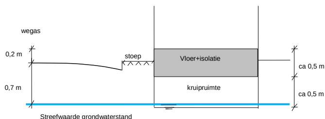
Figuur 12: Schematische weergave streefwaarde grondwaterstand onder kruipruimtebodem bij nieuwbouwwoningen met dikke constructievloeren.
