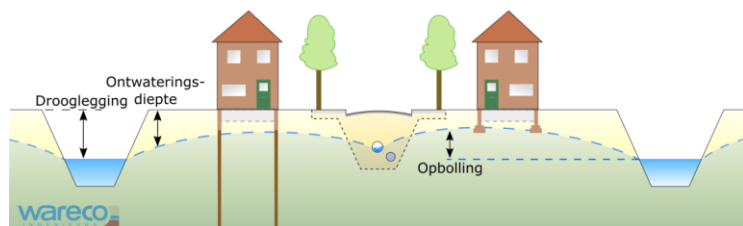
Figuur 13: Voorbeeld van het verloop van de grondwaterstand bij openbaar terrein ten opzichte van particuliere percelen, in zandige gebieden.
