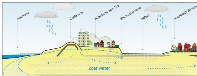
Figuur 9: Schematische doorsnede grondwatersystemen Noordwijk aan Zee tot Noordwijk Binnen (met geel: zand, grijs: kleilagen)
