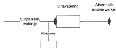
Afbeelding 2: Proces Flow Diagram (PFD) van sliblijn AWZI Noordwijk
