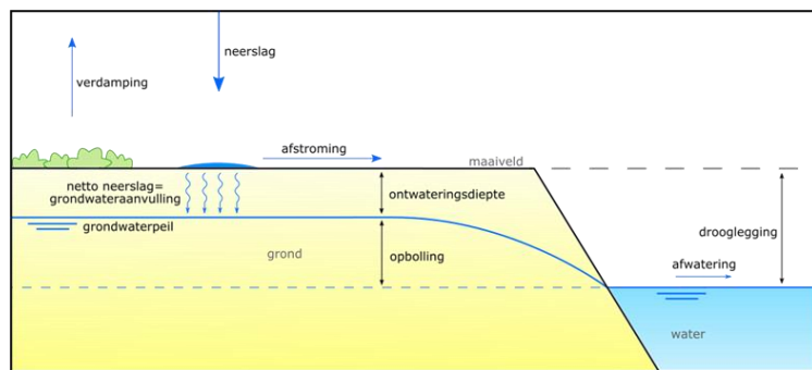
Figuur 15. Schematisatie van enkele hydrologische begrippen.
