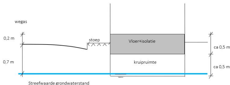
Figuur 18. Schematische weergave streefwaarde grondwaterstand onder kruipruimte bodem bij nieuwbouwwoningen met dikke constructievloeren.
