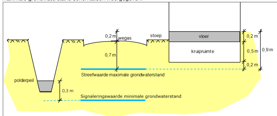
Figuur 17. Streefwaarde voor maximale grondwaterstanden beneden het straatpeil ten opzichte van de kruipruimte en signaleringswaarde voor de minimale grondwaterstand beneden het oppervlaktewaterpeil, in bestaand bebouwd gebied met veenlagen (met een gangbaar profiel van de openbare weg ten opzichte van de woninghoogte).
