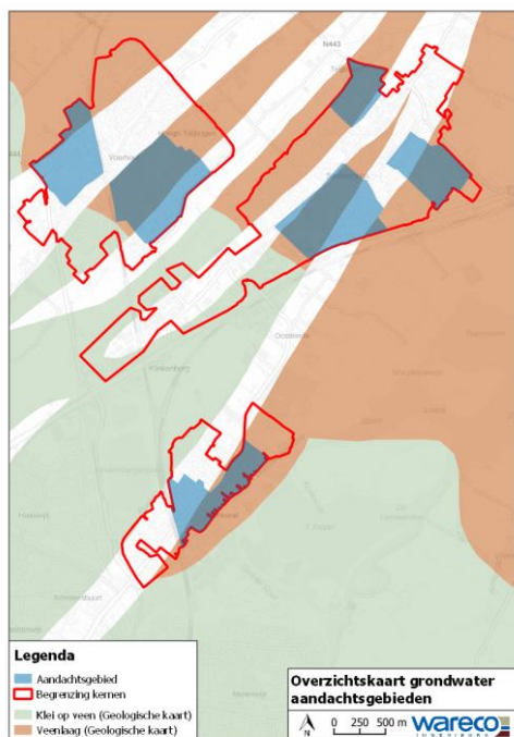
Figuur 16. Overzichtskaat van grondwateraandachtsgebieden in Teylingen. In blauw de aandachtsgebieden voor hoge grondwaterstanden, in groen/oranje de gebieden die kwetsbaar zijn bij het voorkomen van lage grondwaterstanden
