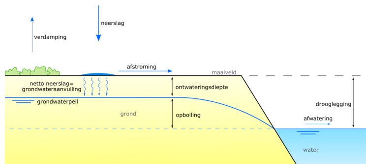
Figuur 8: Principeschets van hydrologische begrippen
