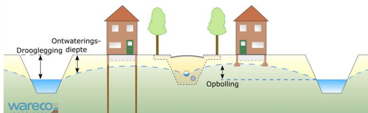
Figuur 20. Voorbeeld van het verloop van de grondwaterstand bij openbaar terrein ten opzichte van particuliere percelen, in zandige gebieden.
