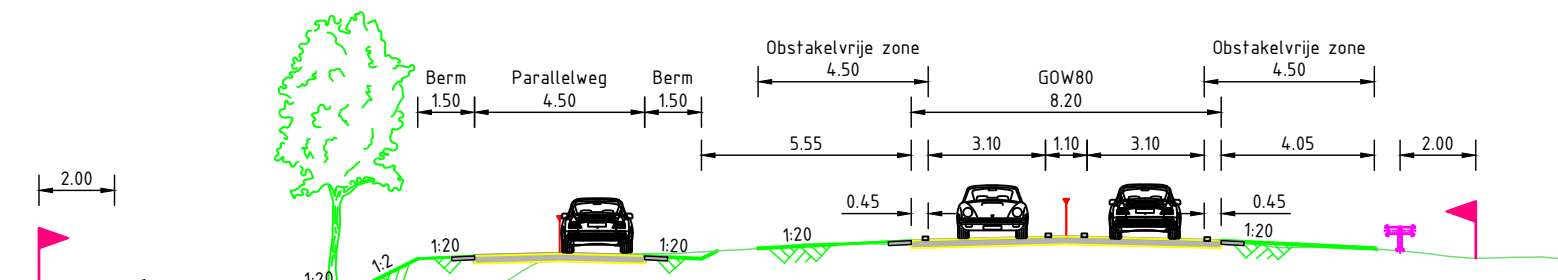
Dwarsprofiel A-A, GOW 80km/h met parallelweg
