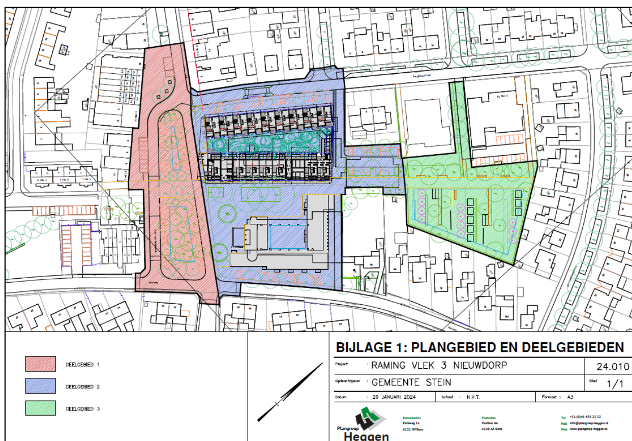
Figuur1: Stedenbouwkundige schets
