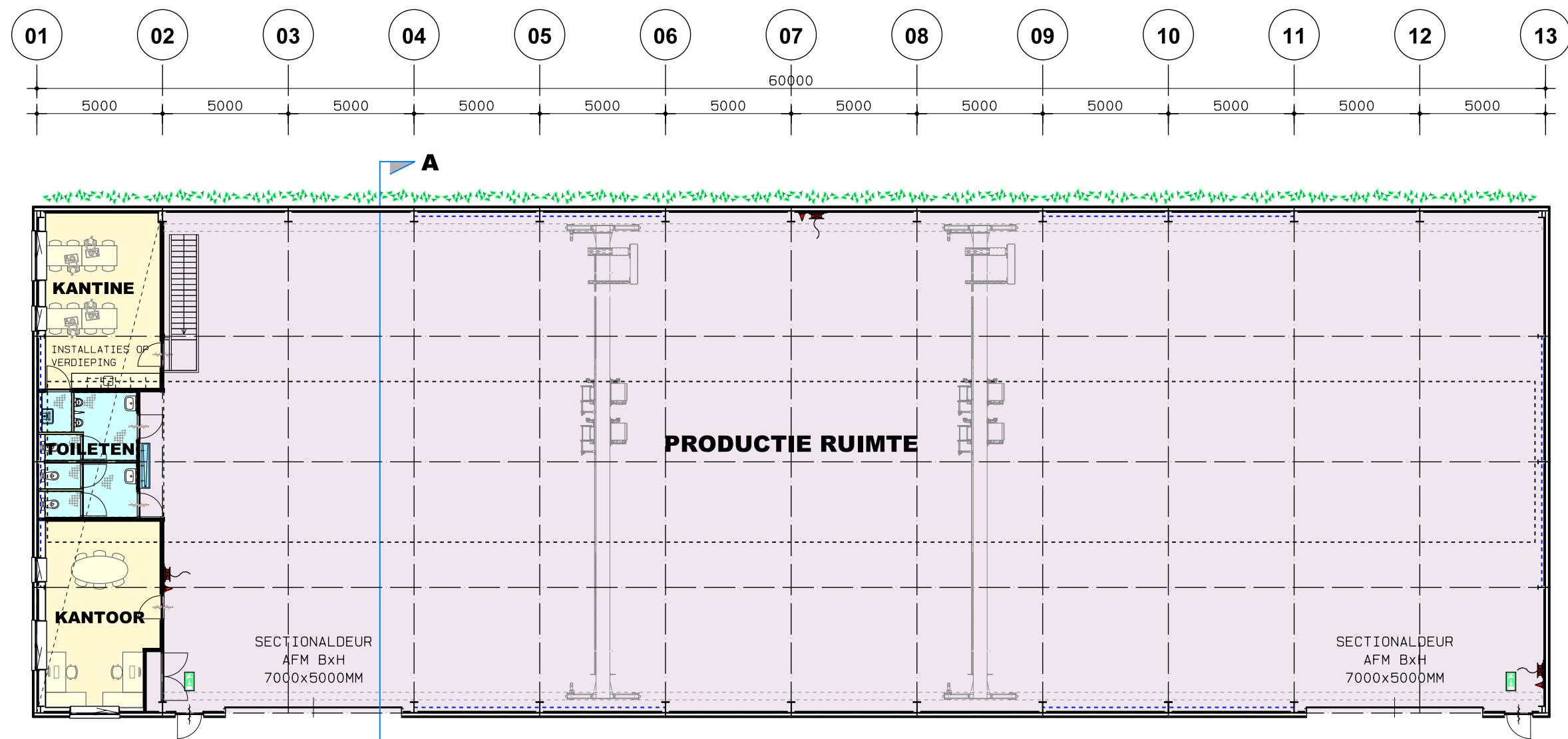
PLATTEGROND
