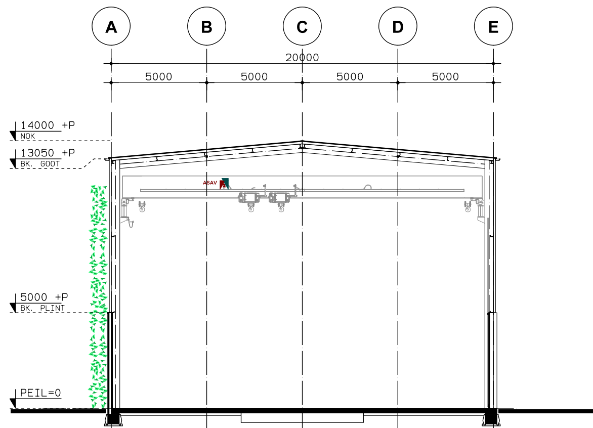
DOORSNEDE A-A
