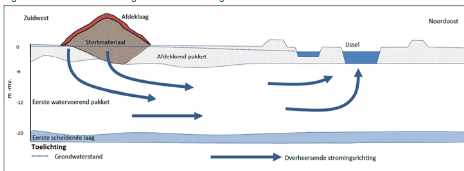
Figuur 1: Dwarsdoorsnede grondwaterstroming
