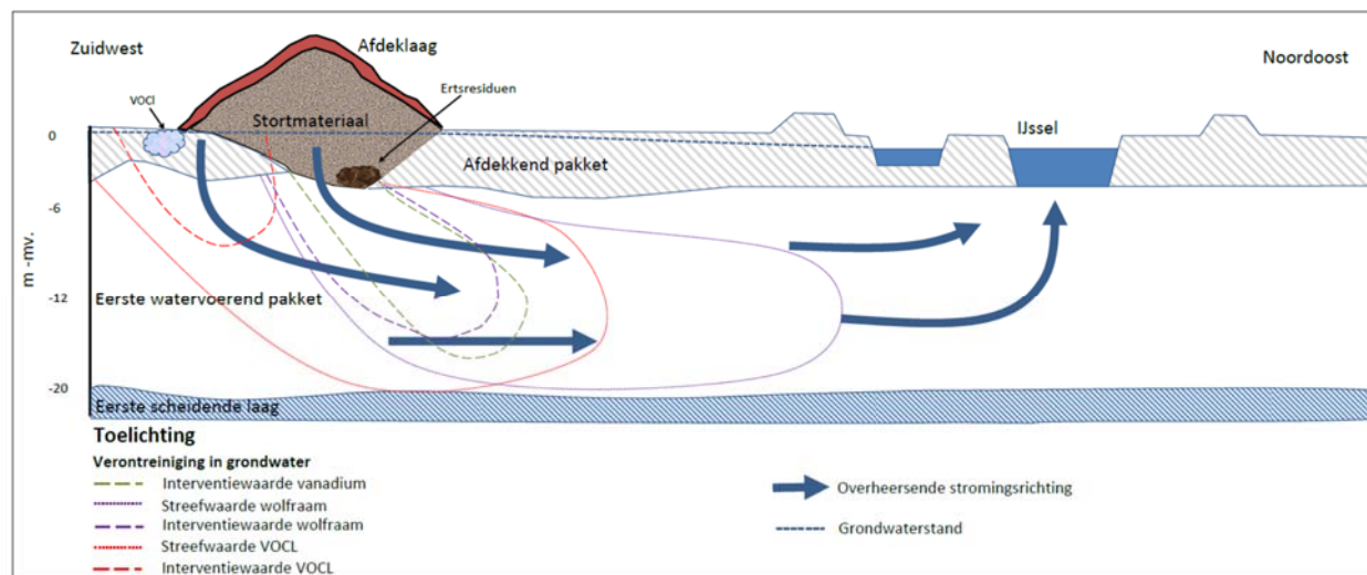
Figuur 2: Dwarsdoorsnede met grondwaterverontreiniging
