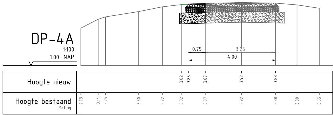
4.3 - Nieuwe situatie - B3 - Sint Bavodijk (fietsstraat)
