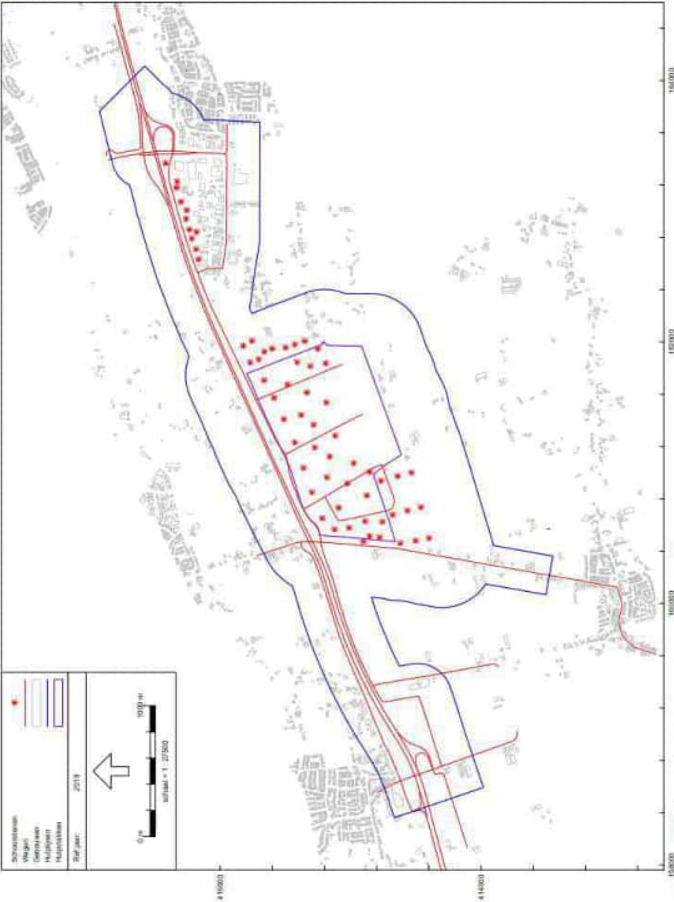
100000 Luchtkwaliteit - 8 TACOS - rekenmodel luchtkwaliteit - alternatief 2 - Gemeente V4.10
