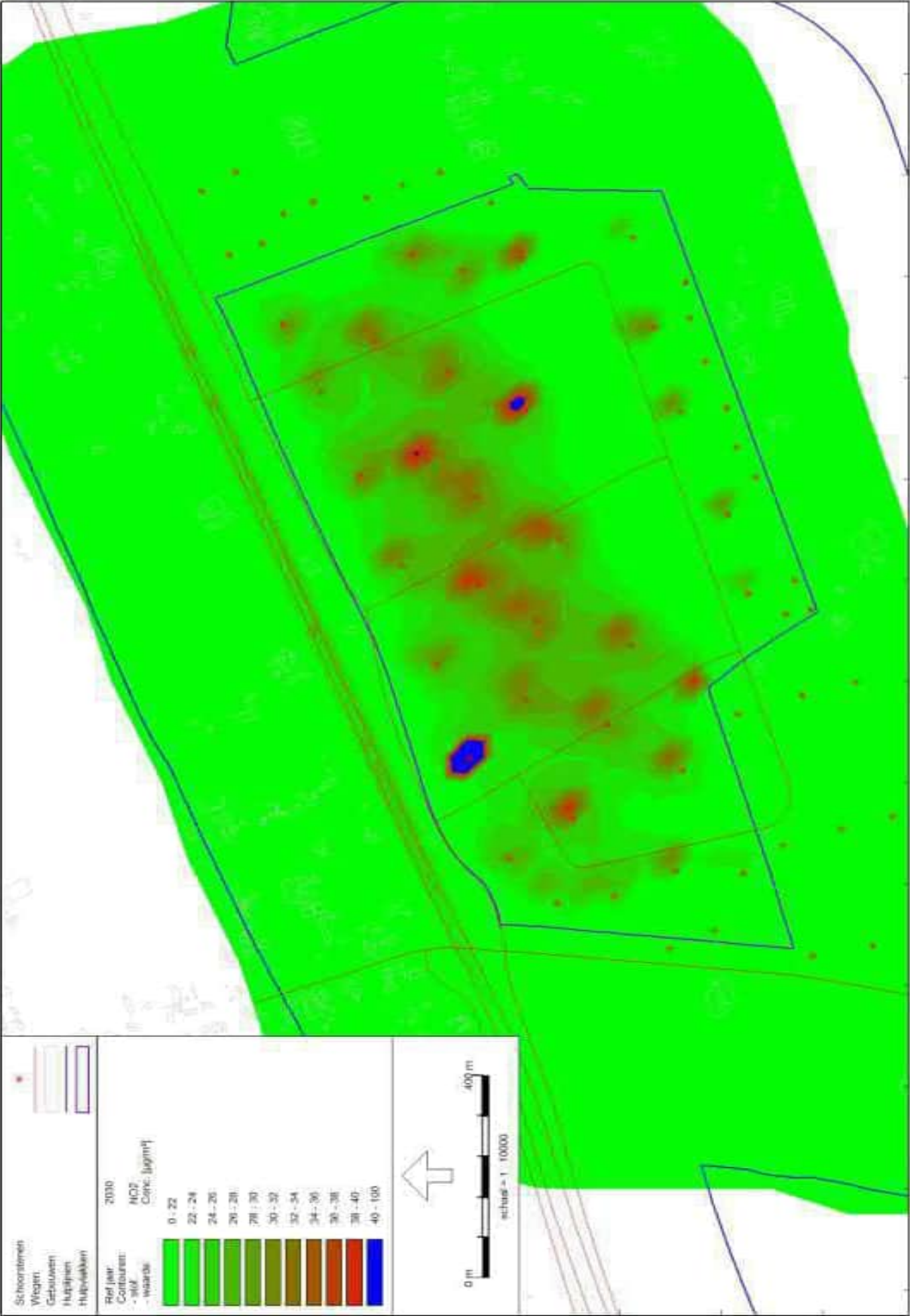
Luftkwaliteit - STACOS (rekenmodellen luchtkwaliteit 2025 - alternatief 3) - Geversden V4.30 Alternatief 3 - Contouren jaargemiddelde concentratie NO2 (2030)
