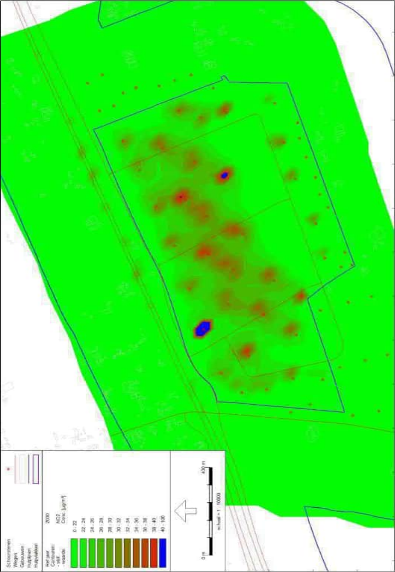
Luftkwaliteit - STACOS (rekenmodellen luchtkwaliteit 2030 - alternatief 4) - Georeferentie V4.30 Alternatief 4 - Contouren jaargemiddelde concentratie NO2 (2030)
