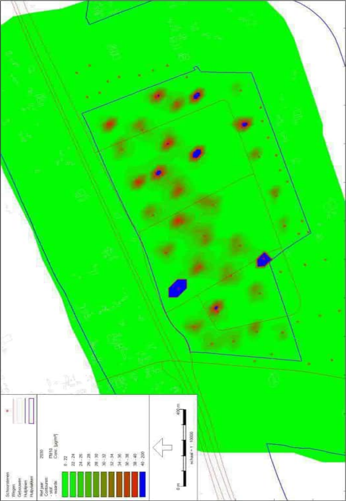
Luchtkwaliteit - STACOS (rekenmodellen luchtkwaliteit 2029 - alternatief 3) - Georeferentie V4.30 Alternatief 3 - Contouren jaargemiddelde concentratie PM10 (2030)
