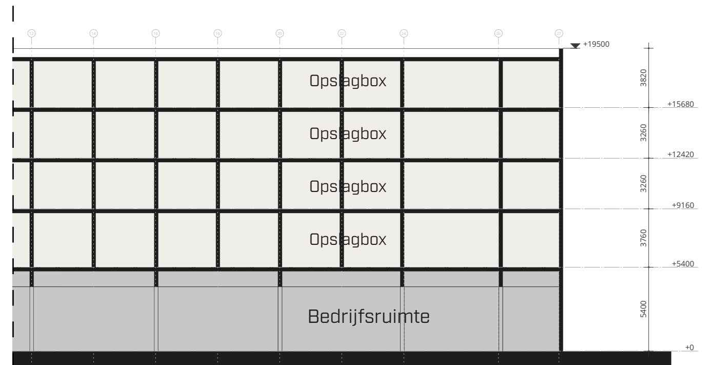
Doorsnede gebouw 2
