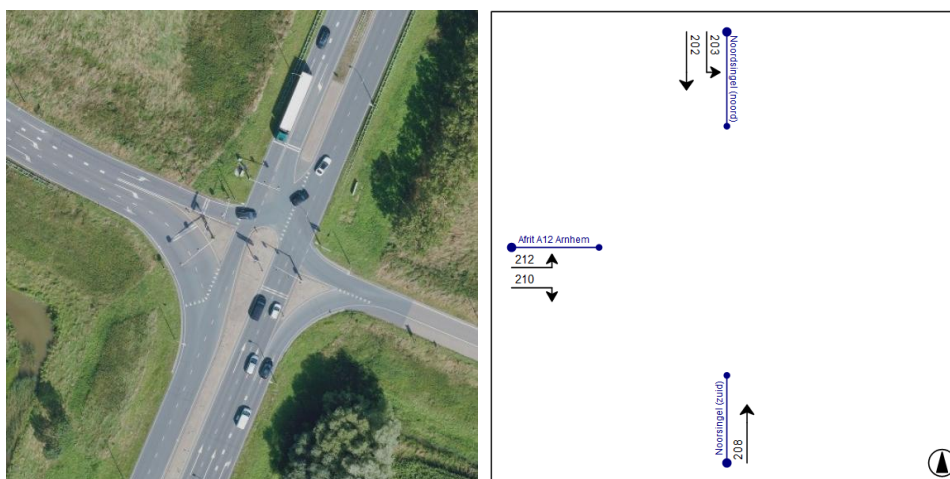
Figuur 2: Vormgeving kruispunt Noordsingel – zuidelijke aansluiting A12
