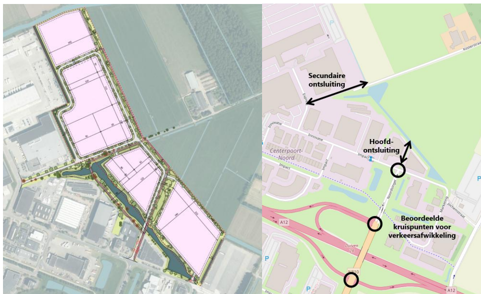
Figuur 1: Stedenbouwkundig plan Centerpoort-Noord II (links) en ontsluiting verkeer (rechts)
