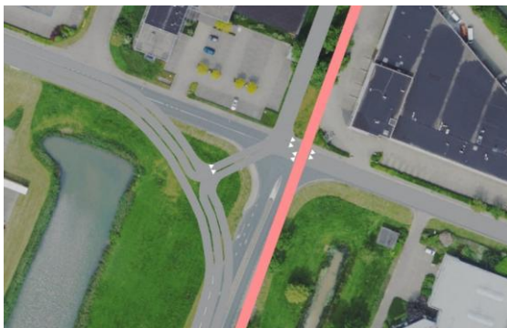
Figuur 10: Voorrangskruispunten met fietsoversteek en aanvullend een bypass
