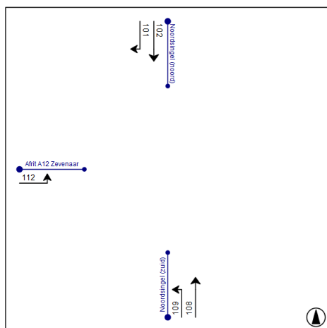
Figuur 4: Alternatieve VRI-vormgeving met aparte signaalgroep voor linkafslaand verkeer
