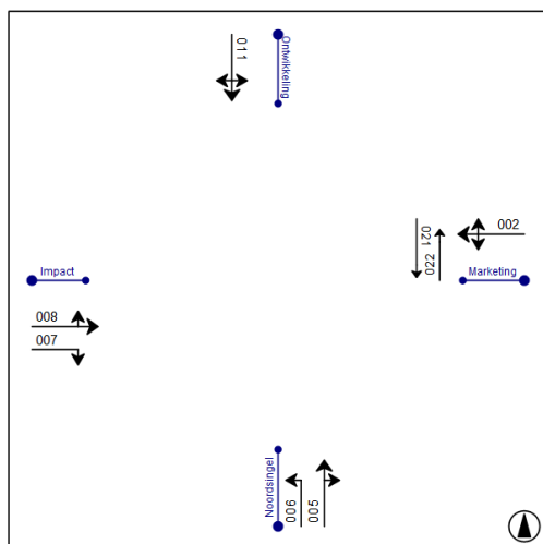
Figuur 8: Vormgeving met verkeerslichten
