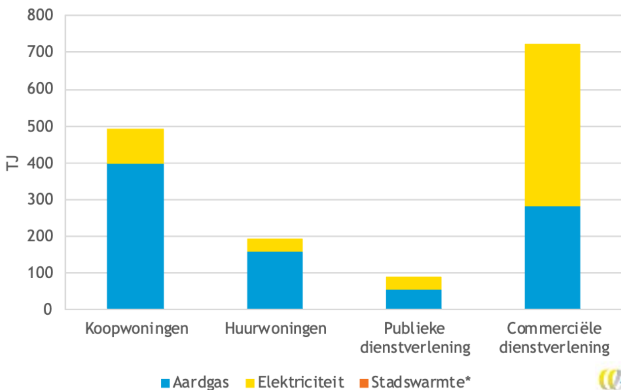
Figuur 20 - Energieverbruik in de gebouwde omgeving
