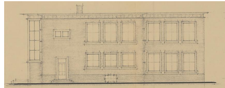
Rechterzijgevel op bouwtekening uit 1953. Bron: RHCe.
