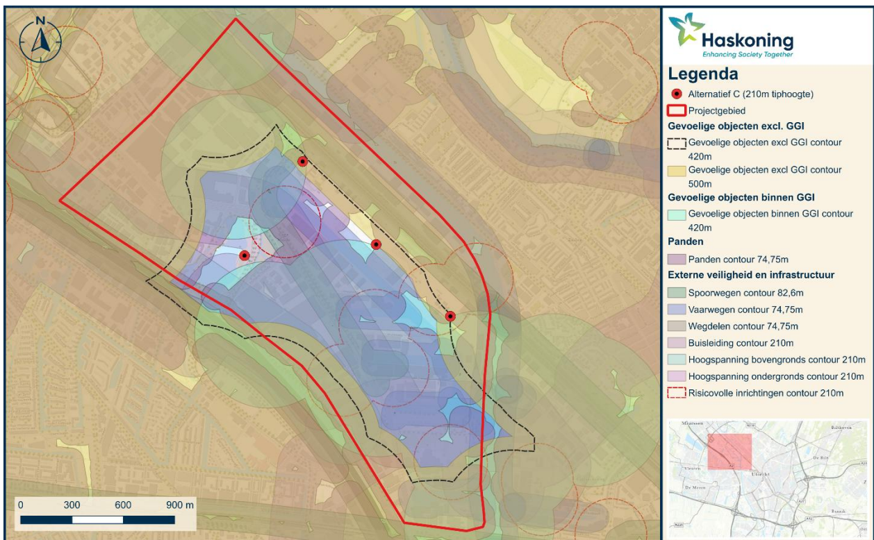
Figuur 3.9 Alternatief C (tiphoogte 210 meter) inclusief belemmeringen
