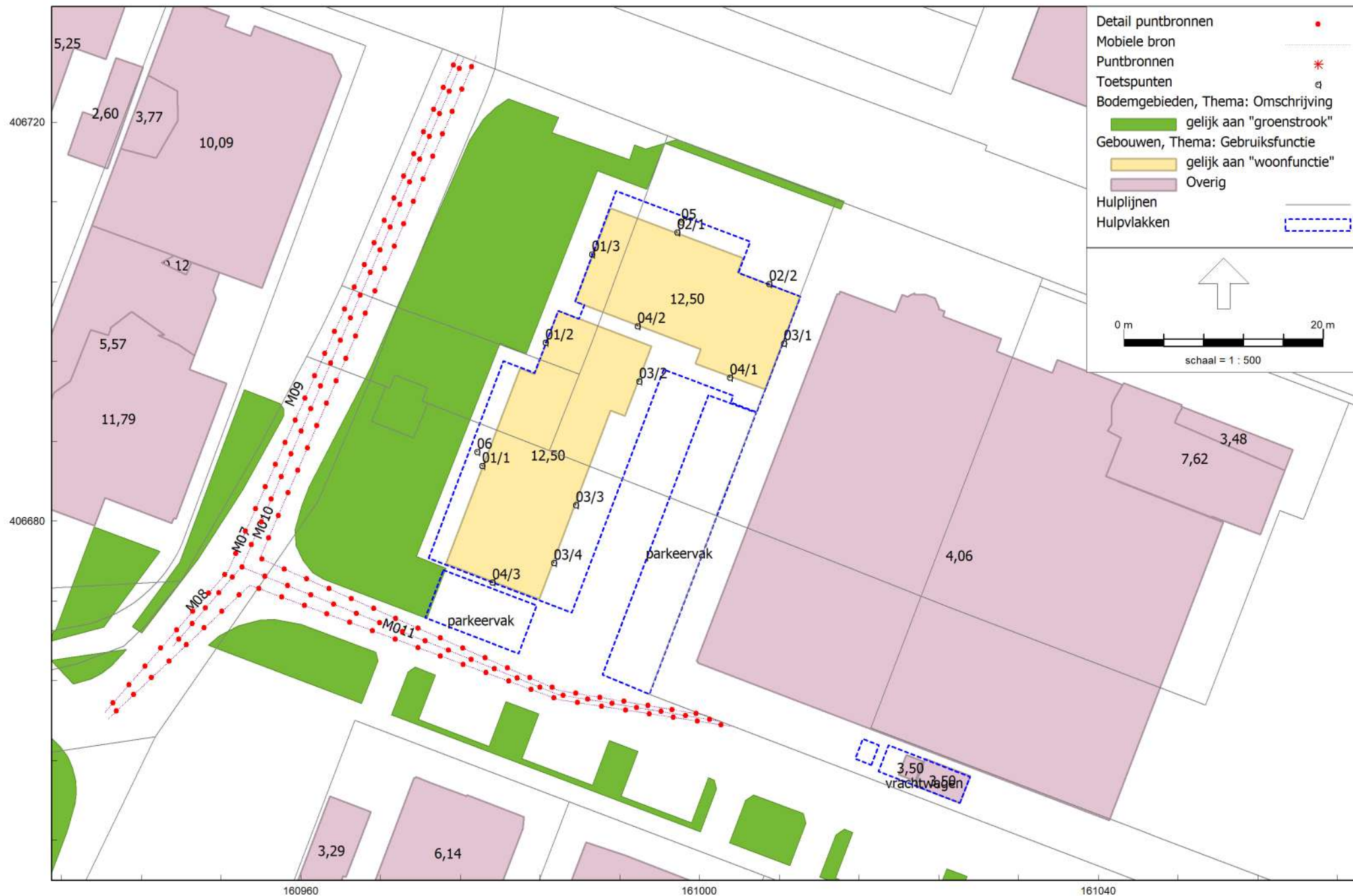
Situatie met geluidbronnen verkeer openbare weg
