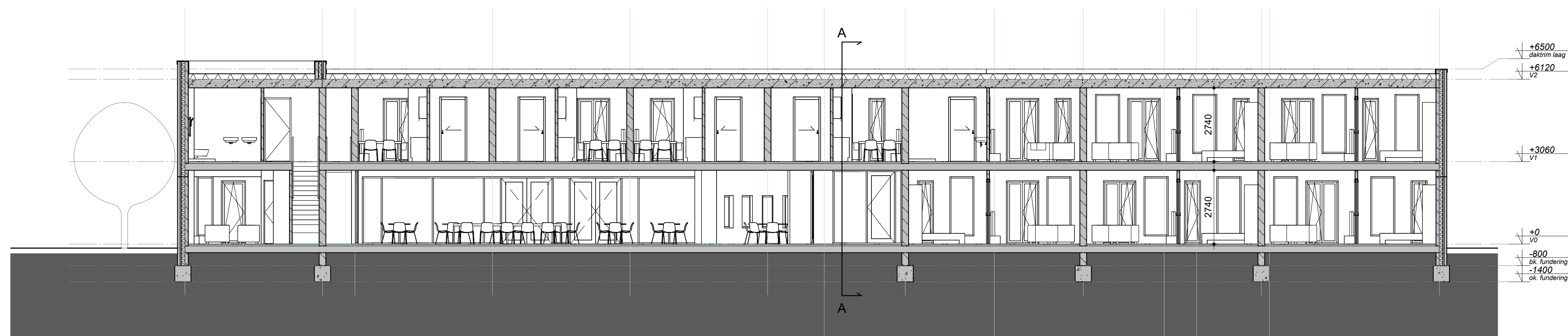
doorsnede B-B
