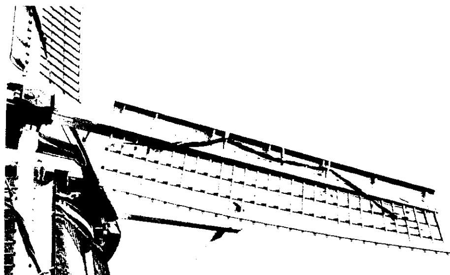
Afb. 13-4. Wiek van de korenmolen 'De Vriendschap' te Weesp. Fokwiel uitgerust met remkleppen en steekborden.
