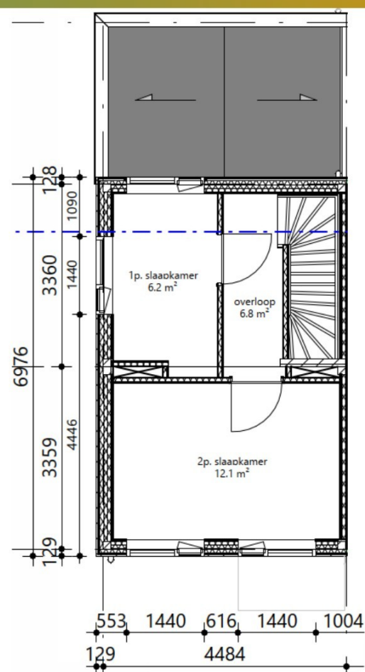
tweede verdieping
