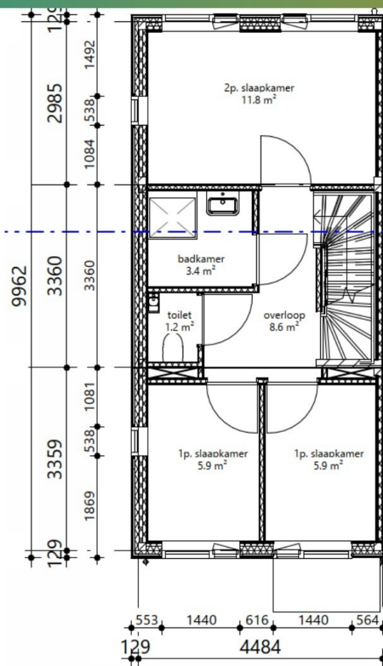
eerste verdieping
