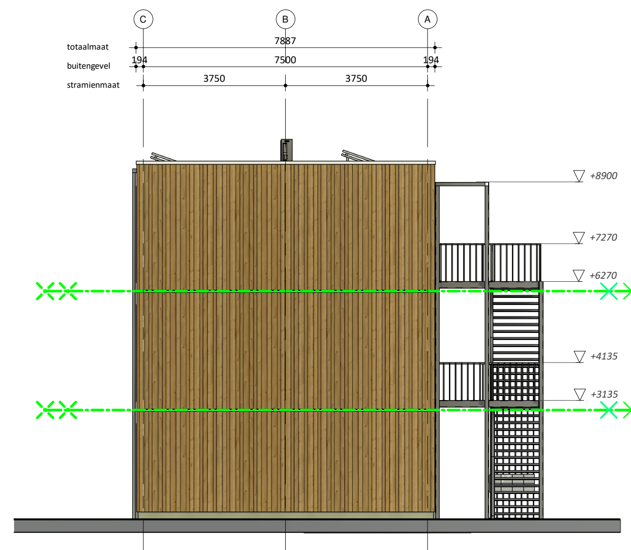
Linkergevel
