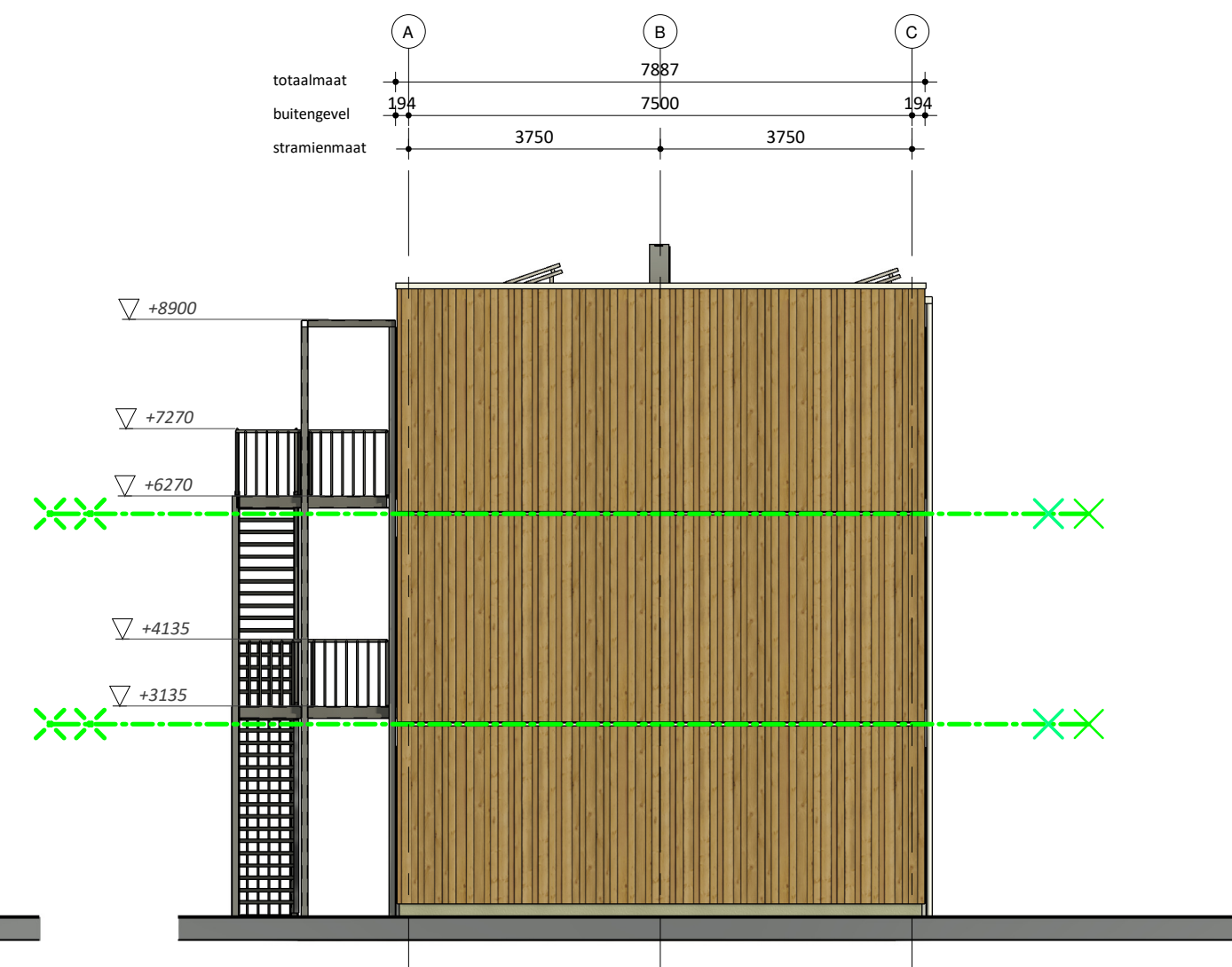
Rechtergevel
