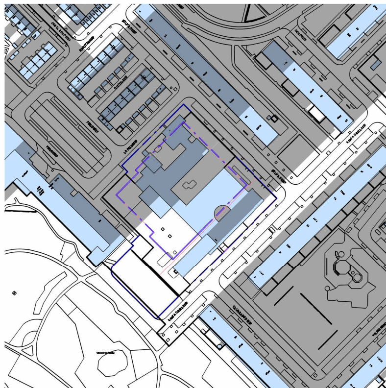
21 december 16.00 - bestand
