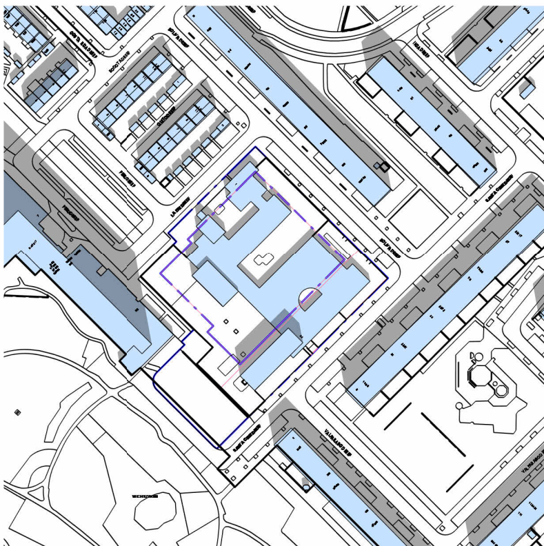
21 september 12.00 - bestand
