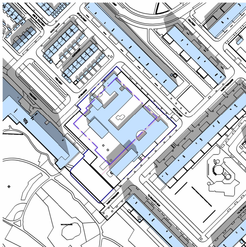
21 maart 12.00 - bestand
