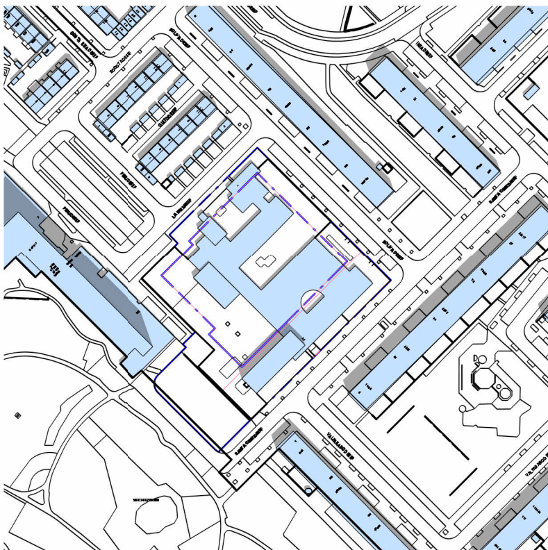
21 juni 12.00 - bestaand
