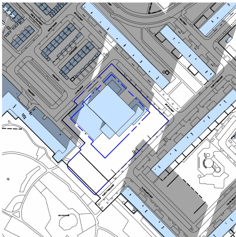
21 december 14.00 - nieuw
