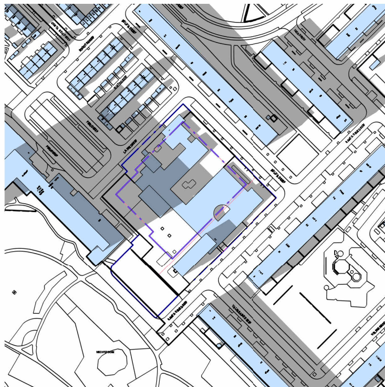
21 september 16.00 - bestand
