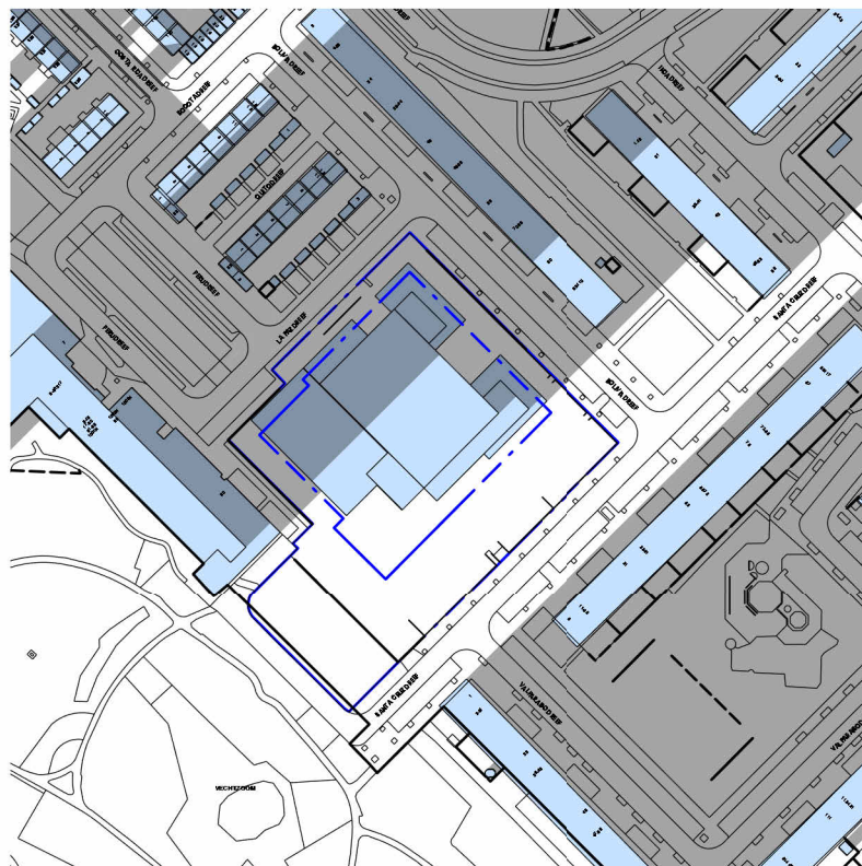
21 december 16.00 - nieuw
