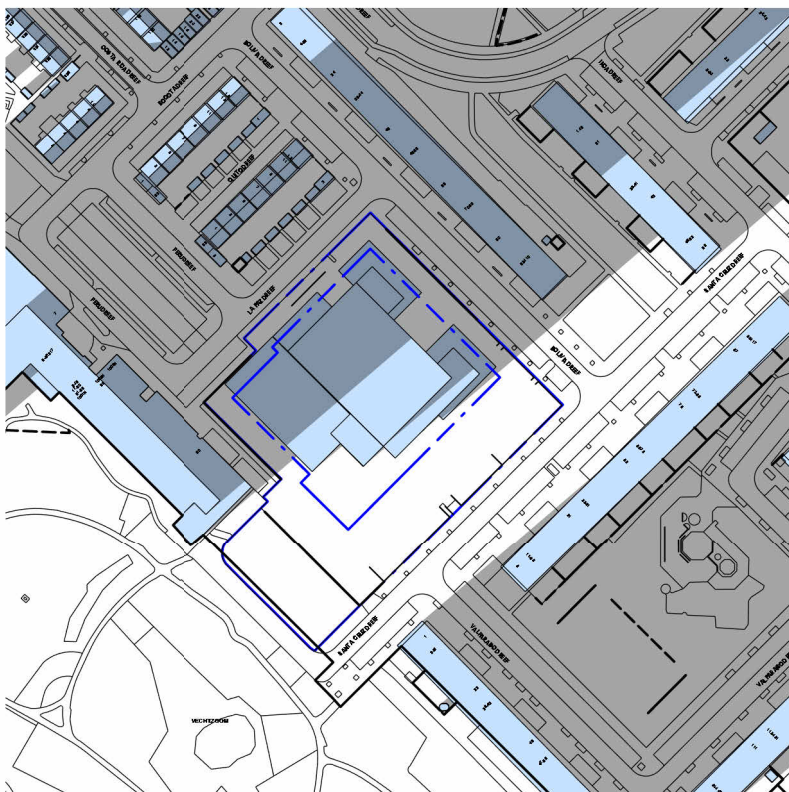
21 december 18.00 - nieuw
