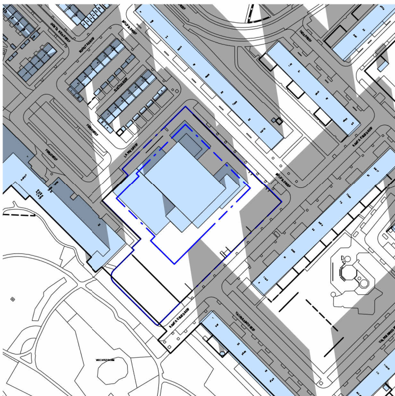
21 december 12.00 - nieuw
