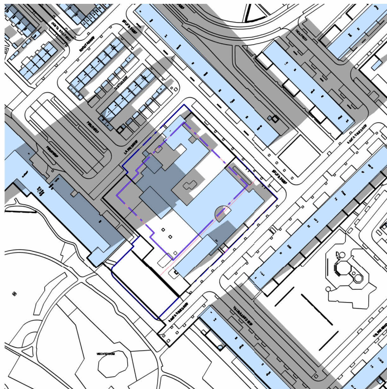
21 maart 16.00 - bestand
