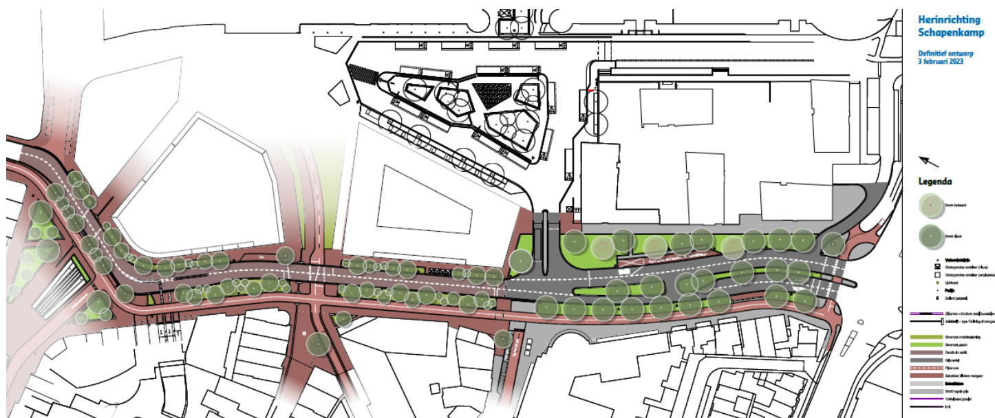
Afbeelding 1 – Definitief ontwerp Schapenkamp
