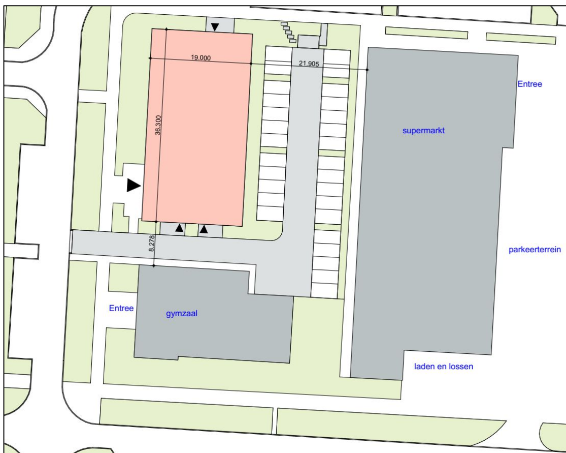
Figuur 9. Situatieschets nieuwbouw en omliggende bedrijvigheid.
