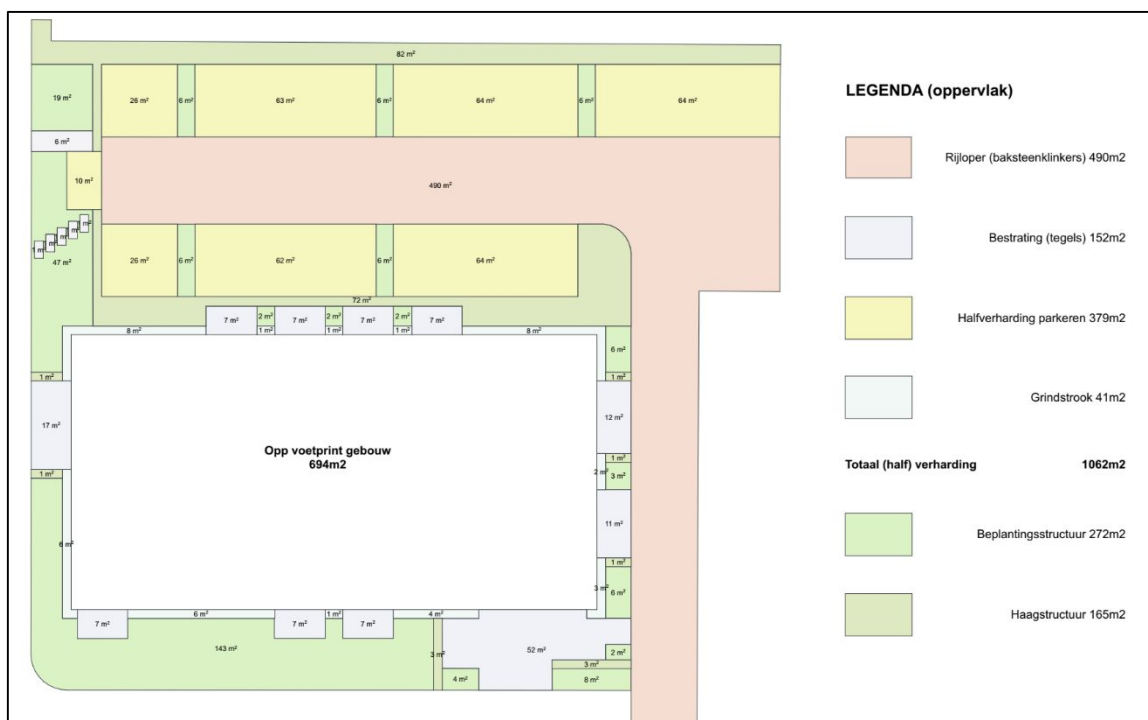
Figuur 14. voorlopige terreinindeling en verharding (bron: CH|NL) .
