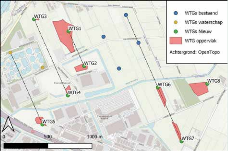
Figuur 4. Scenario 1 wind. De zwarte stippellijnen geven de oriëntatie van de nieuwe windturbines in relatie tot de al bestaande windturbines weer.
