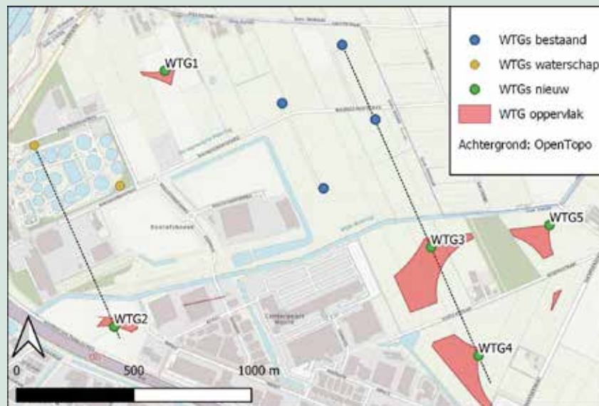
Figuur 8. Scenario 3 wind. De zwarte stippellijnen geven de oriëntatie van de nieuwe windturbines in relatie tot de al bestaande windturbines weer.
