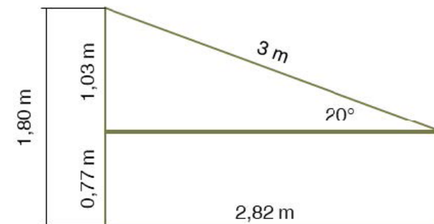
Figuur 3. Zijaanzicht van de zonne-energie opstelling.
