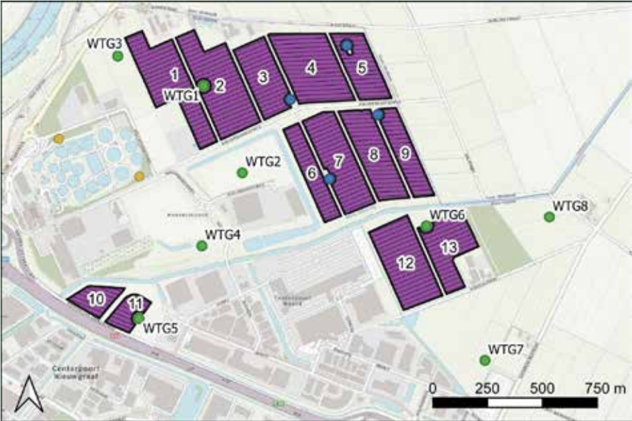
Figuur 5. Scenario 1 met windturbines met afmetingen 120 / 120 m (ashoogte / rotordiameter). De zwarte omlijning geeft de onderhoudspaden langs de randen van de zonnevelden weer.
