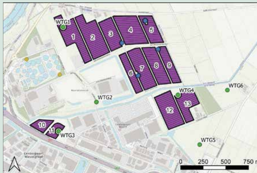
Figuur 7. Scenario 2 met windturbines met afmetingen 140 / 142 m (ashoogte / rotordiameter). De zwarte omlijn geeft de onderhoudspaden langs de randen van de zonnenvelden weer.
