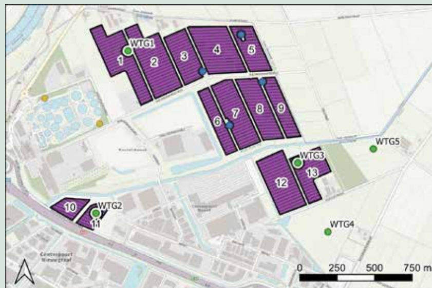
Figuur 9. Scenario 3 met windturbines met afmetingen 160 / 160 m (ashoogte / rotordiameter). De zwarte omlijning geeft de onderhoudspaden langs de randen van de zonnenvelden weer.
