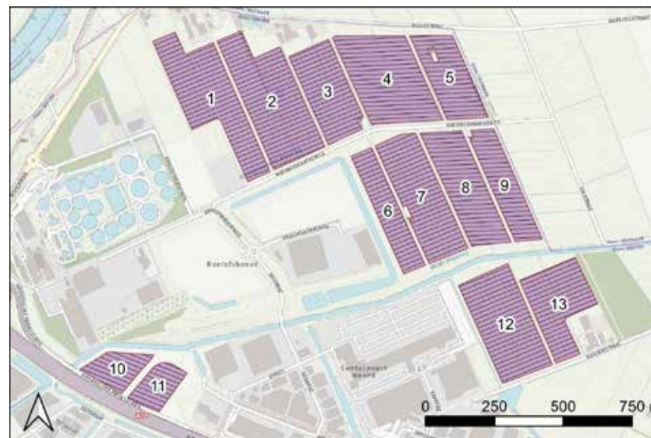
Figuur 2 De velden die beschikbaar zijn voor zonne-energie. De belijning in de velden geven de oriëntatie van de rijen weer.
