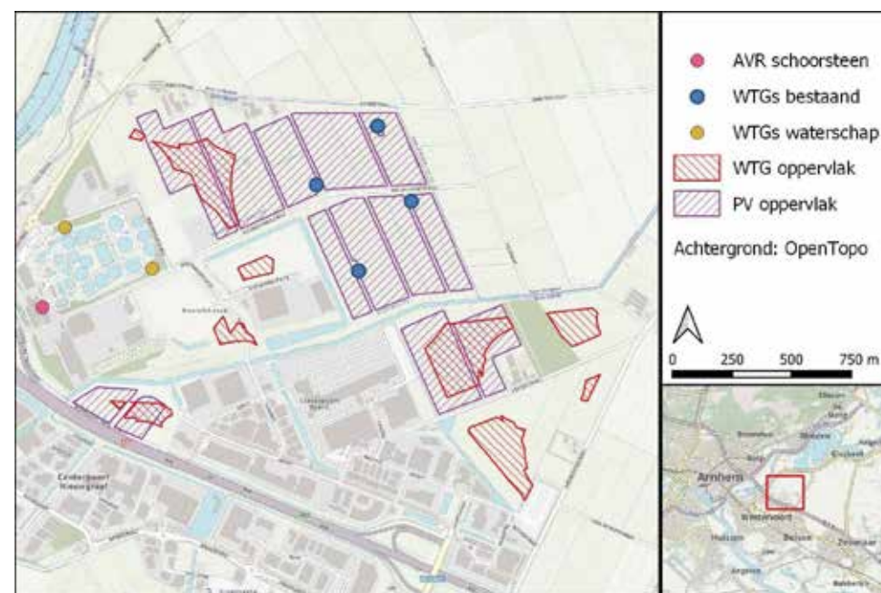
Figuur 1. Locatieoverzicht met beschikbare oppervlakten voor zon en wind. WTG staat voor windturbinegenerator. De AVR schoorsteen is de schoorsteen van het afvalverwerkingsbedrijf
