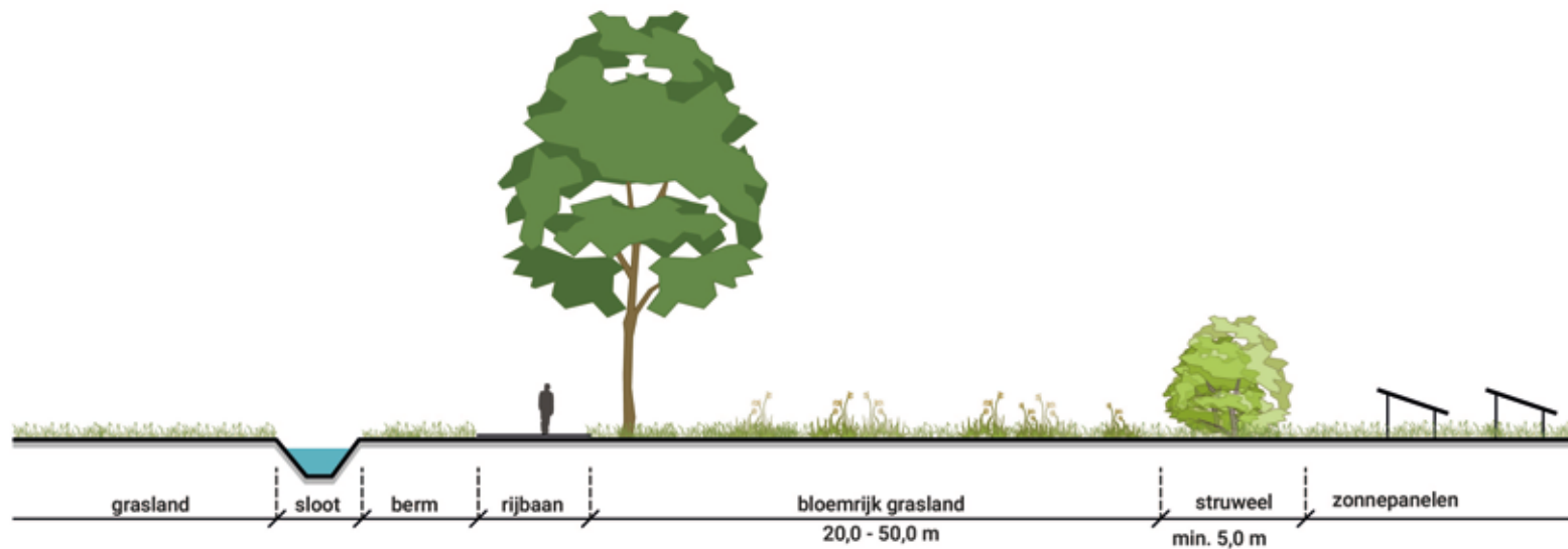
Locatie principeprofiel
