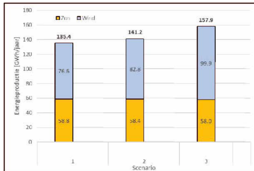
Figuur 10. Totale energieproductie van de scenario's.
