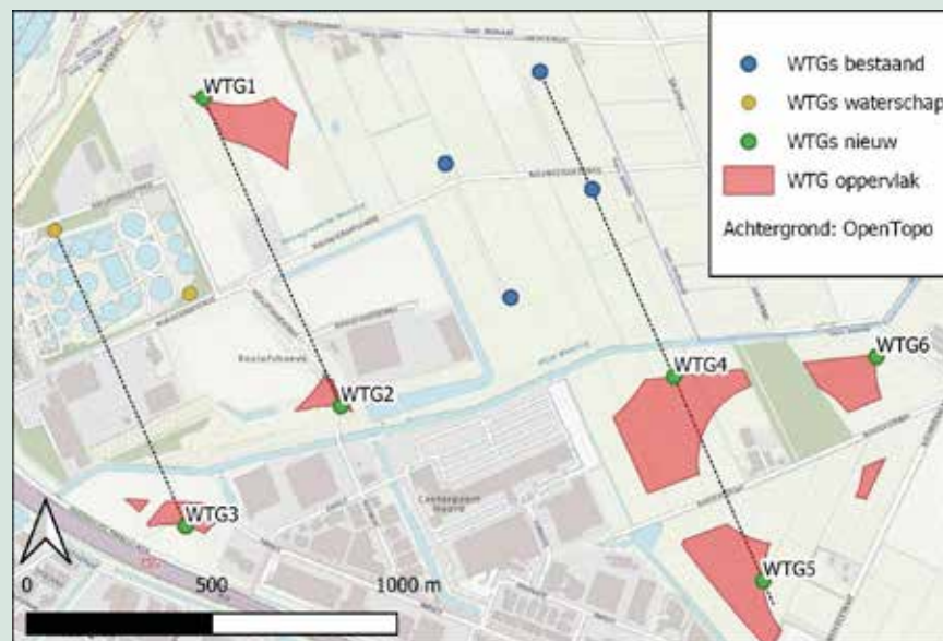
Figuur 6. Scenario 2 wind. De zwarte stippellijnen geven de oriëntatie van de nieuwe windturbines in relatie tot de al bestaande windturbines weer.
