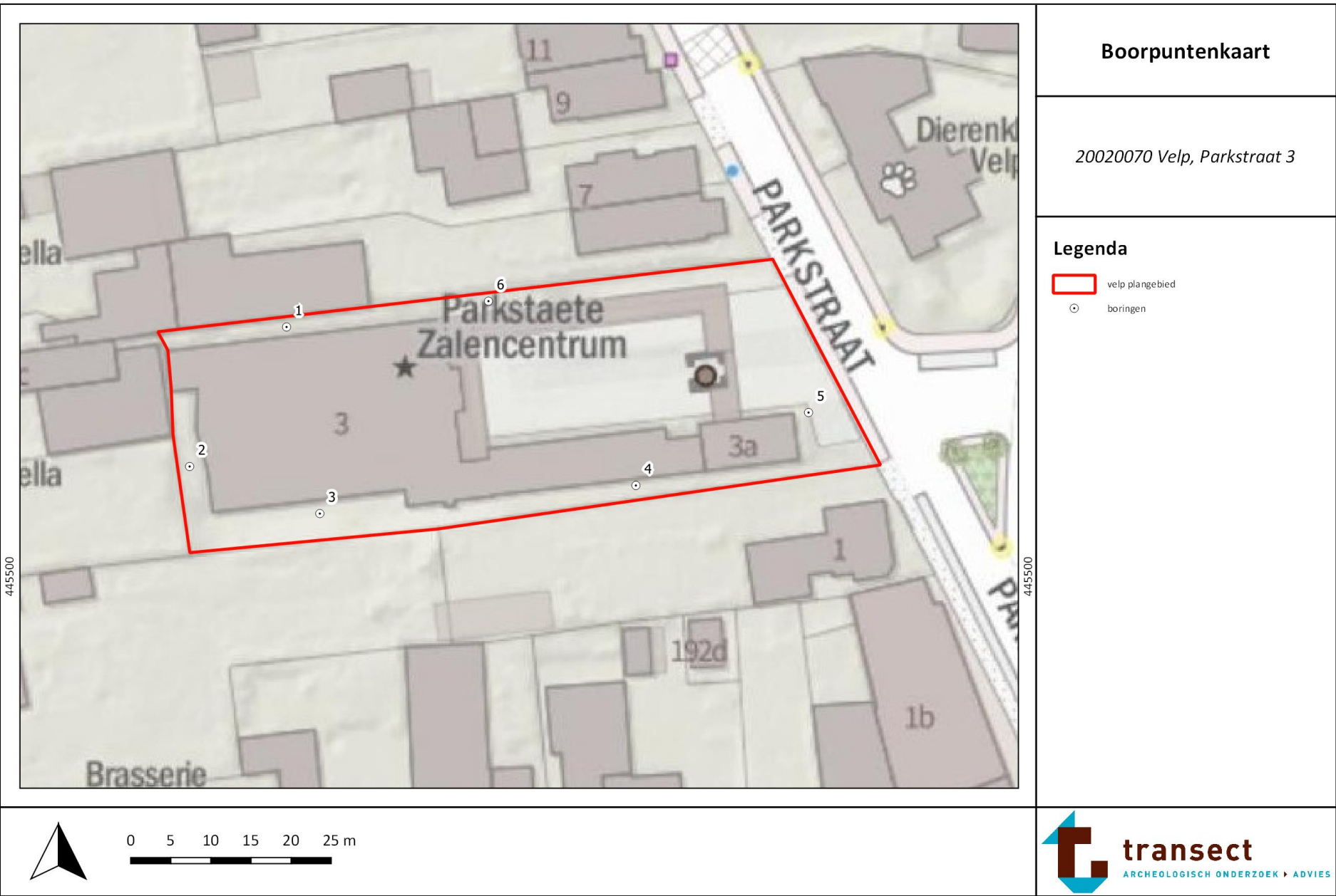
Bijlage 6: Boorpuntenkaart
