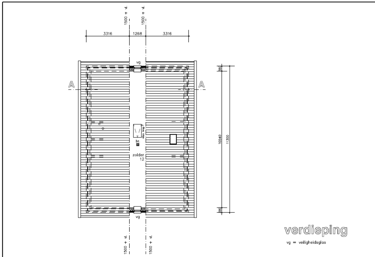
Figuur 2.10. Zolderverdieping toekomstige bedrijfswoning (bron: Accent Bouw Wonen B.V)
