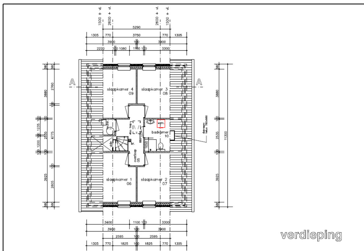
Figuur 2.9. Eerste verdieping toekomstige bedrijfswoning (bron: Accent Bouw Wonen B.V)
