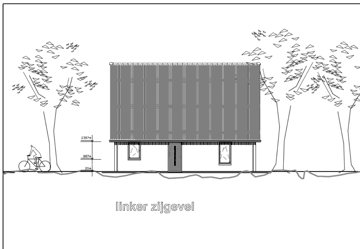
Figuur 2.7. Zijgevel toekomstige bedrijfswoning (bron: Accent Bouw Wonen B.V)
