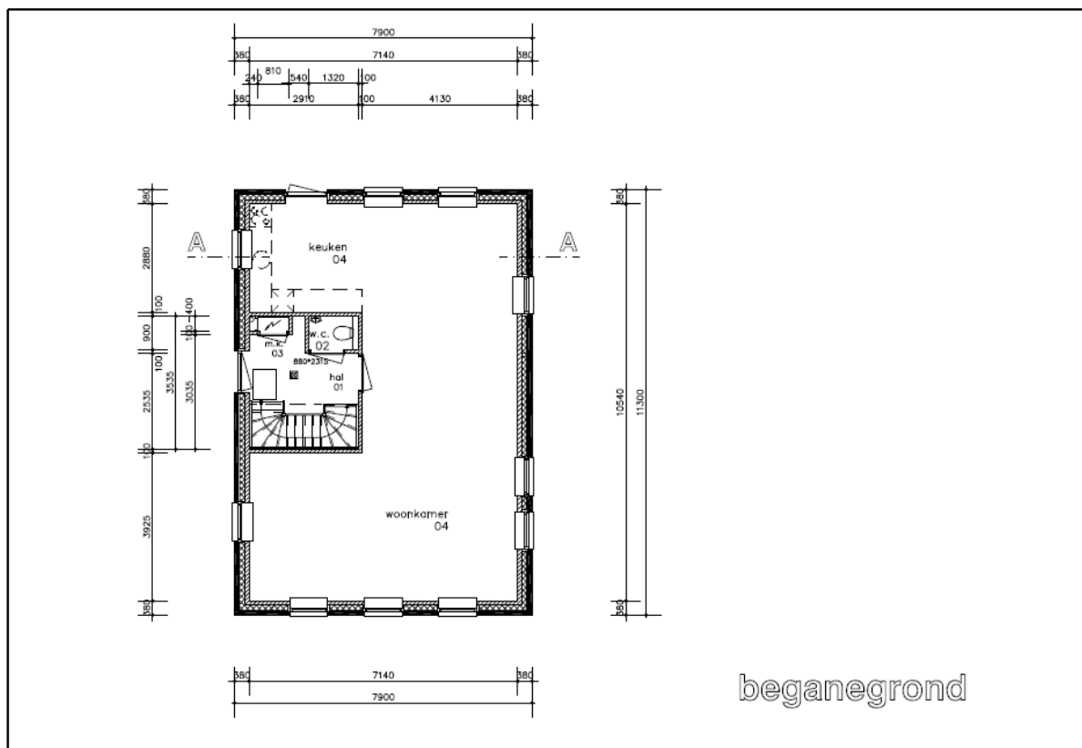
Figuur 2.8. Begane grond toekomstige bedrijfswoning (bron: Accent Bouw Wonen B.V)
