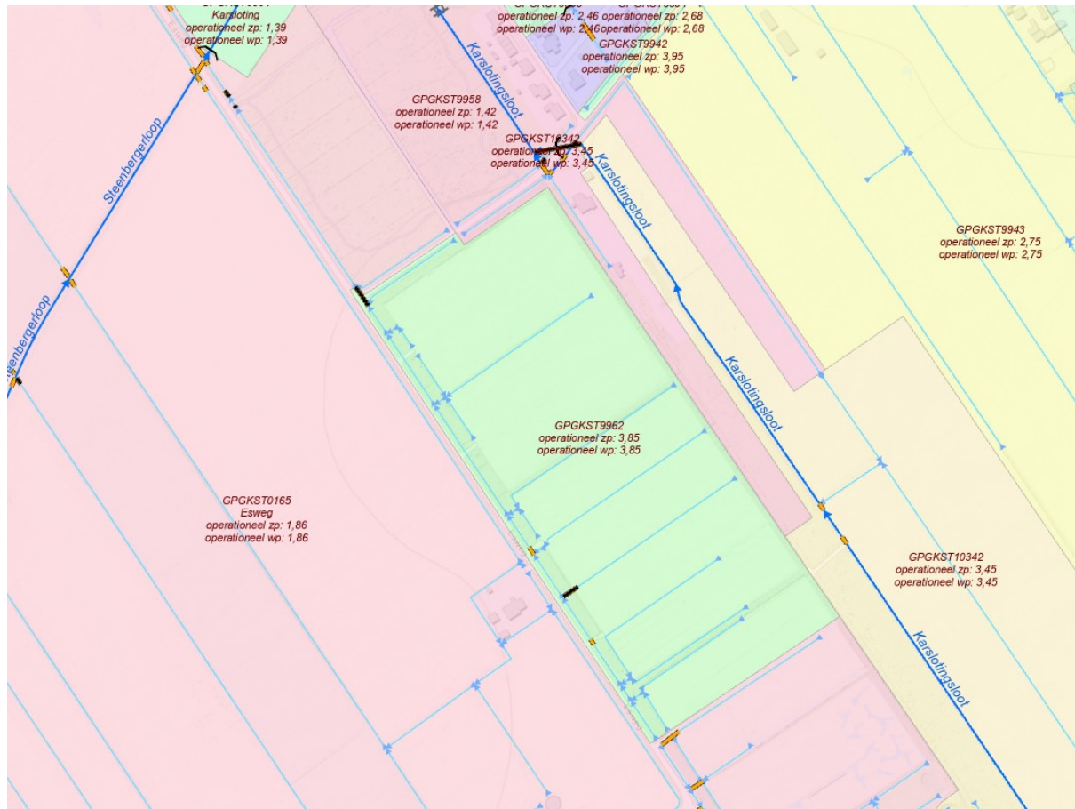
Figuur 4.7. Afwatering projectgebied (bron: Waterschap Noorderzijlvest)
