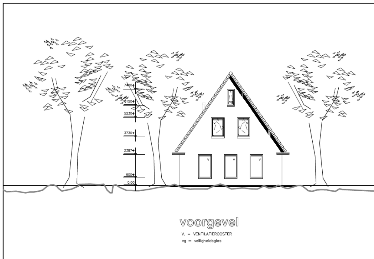
Figuur 2.6. Voorgevel toekomstige bedrijfswoning (bron: Accent Bouw Wonen B.V)
