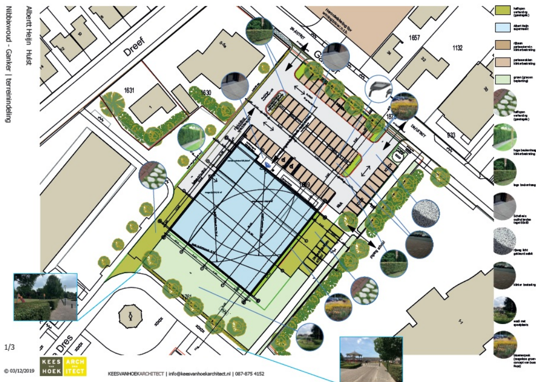
Figuur 2.1 Voorlopig ontwerp terreinindeling toekomstige situatie (bron: Kees van Hoek architect)
