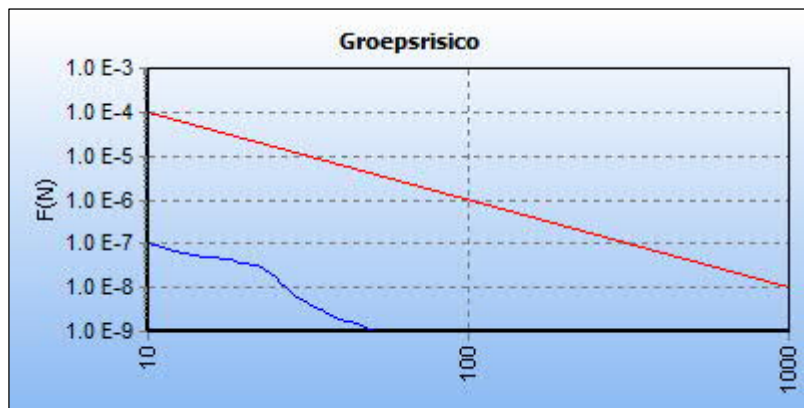
Afbeelding 10: FN-curve huidige situatie A-635
