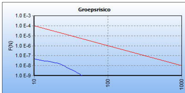
Afbeelding 6: FN-curve huidige situatie A-524
