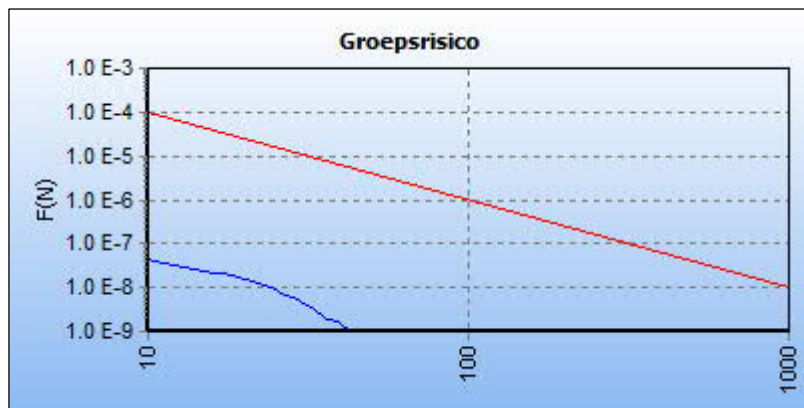
Afbeelding 8: FN-curve huidige situatie A-533
