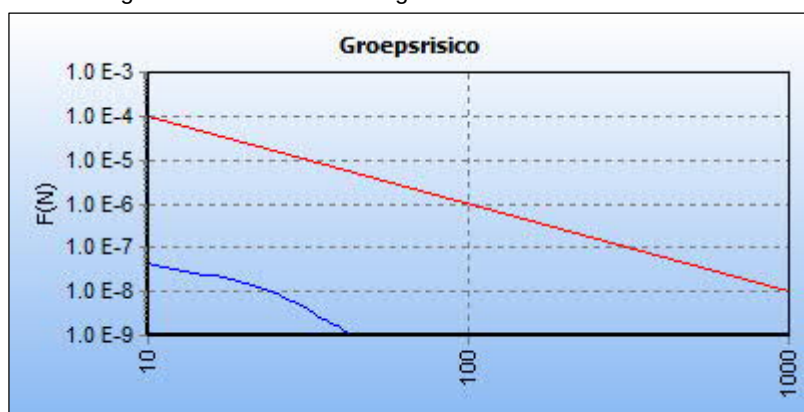
Afbeelding 9: FN-curve toekomstige situatie A-533
