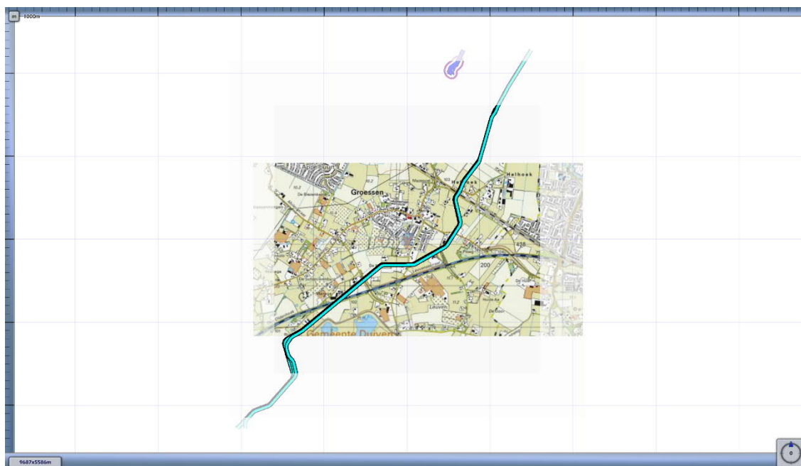
3.4 Figuur 3.4 Plaatsgebonden risico voor 9277_leiding-N-559-10-deel-1 van N.V. Nederlandse Gasunie
