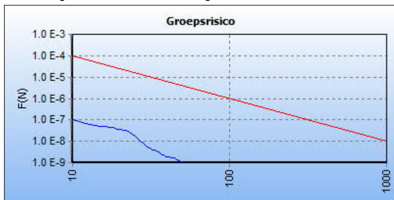
Afbeelding 11: FN-curve toekomstige situatie A-635
