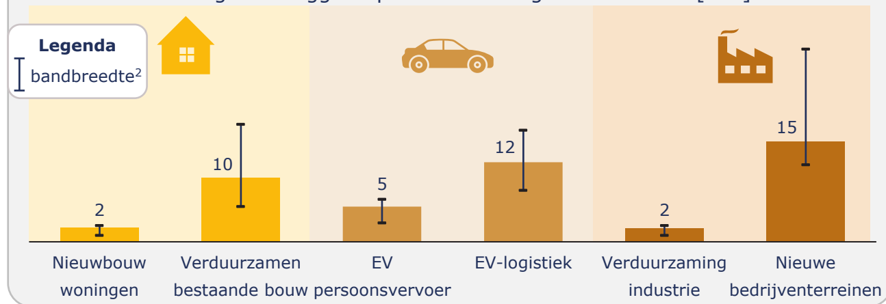
Vermogensvraaggroei per ontwikkeling 1 tot aan 2035 [MW]
