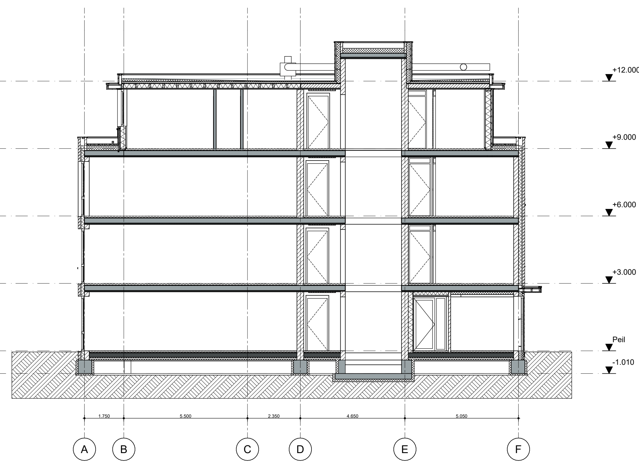
Doorsnede C-C
