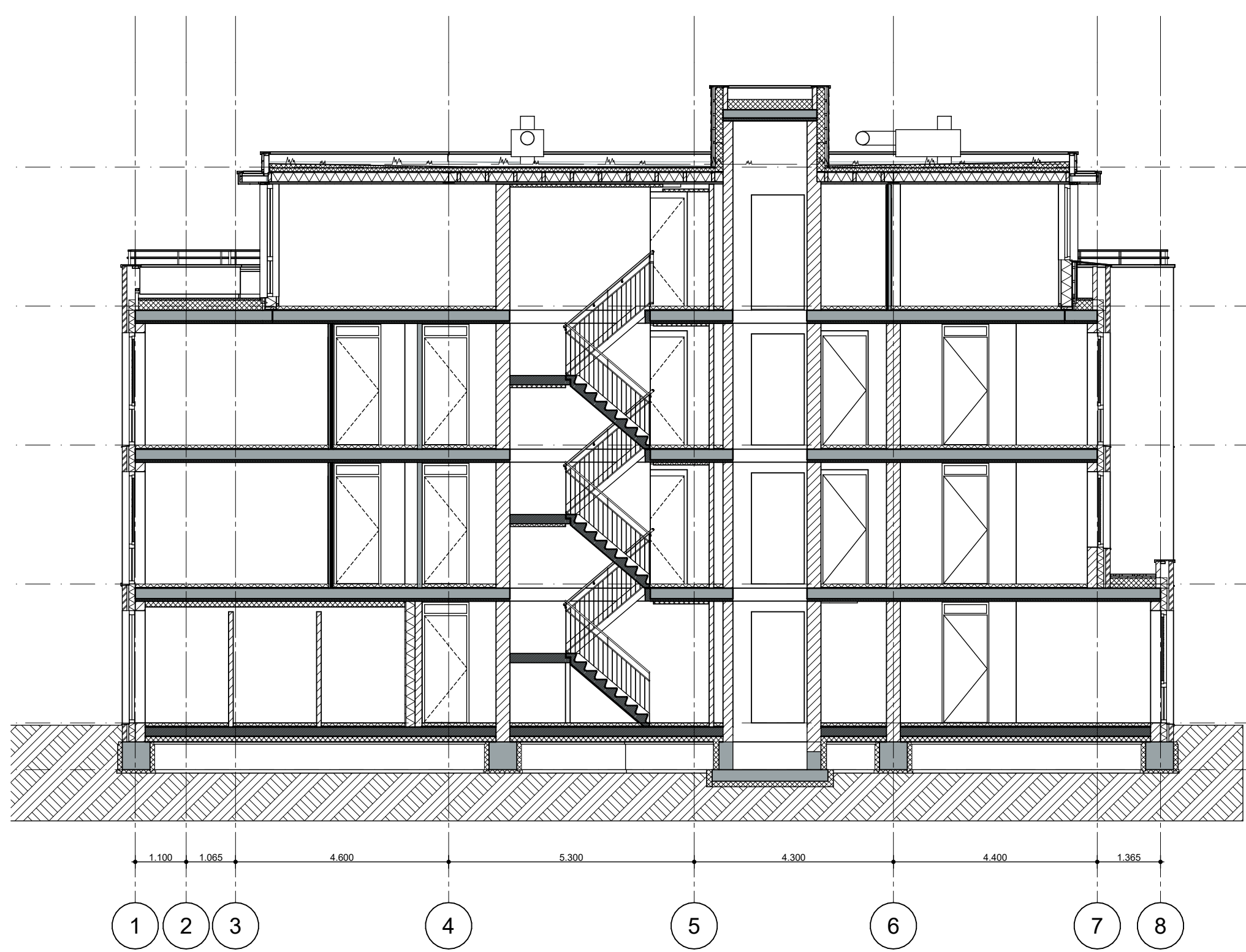
Doorsnede B-B
