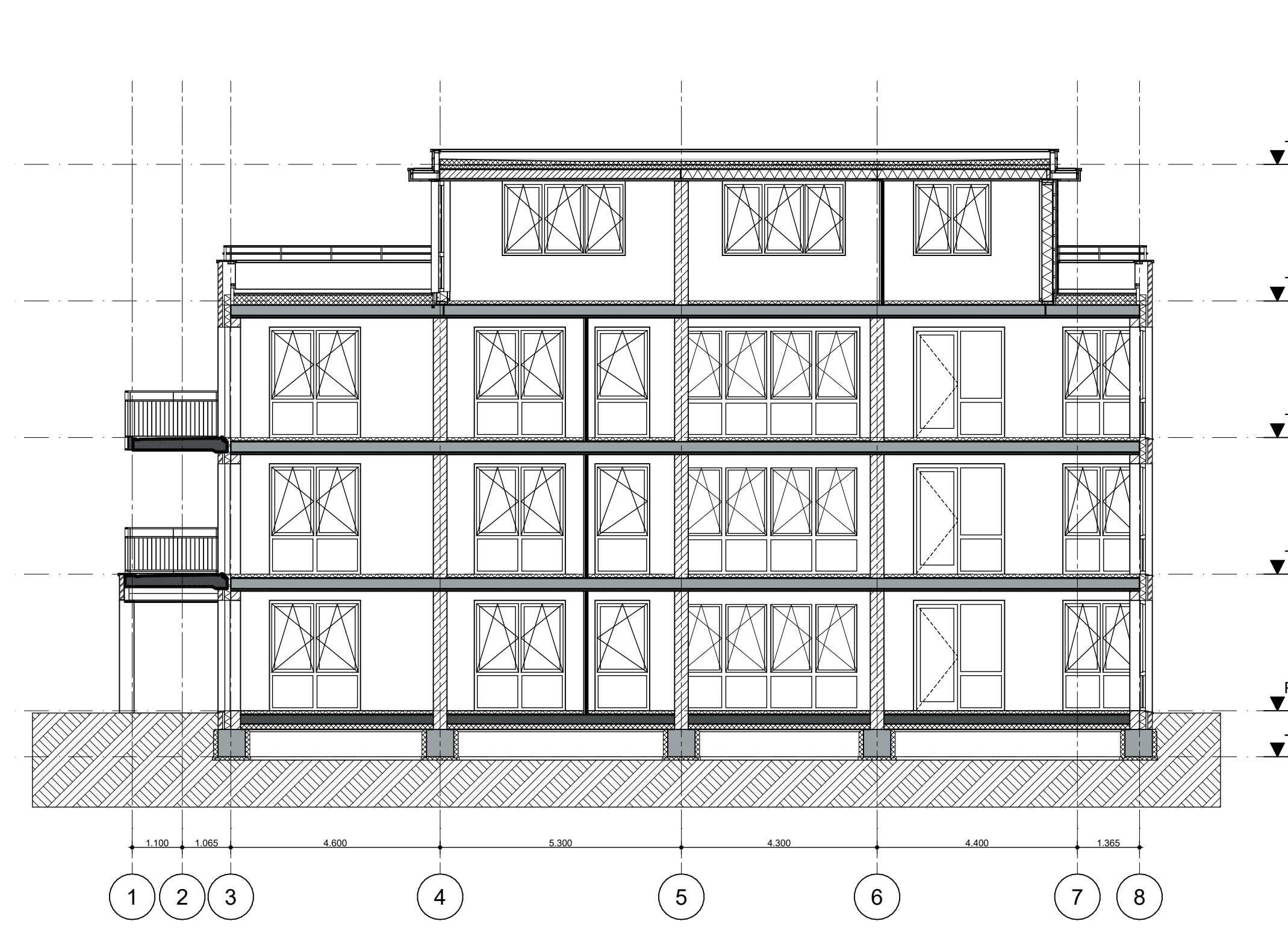
Doorsnede D-D
