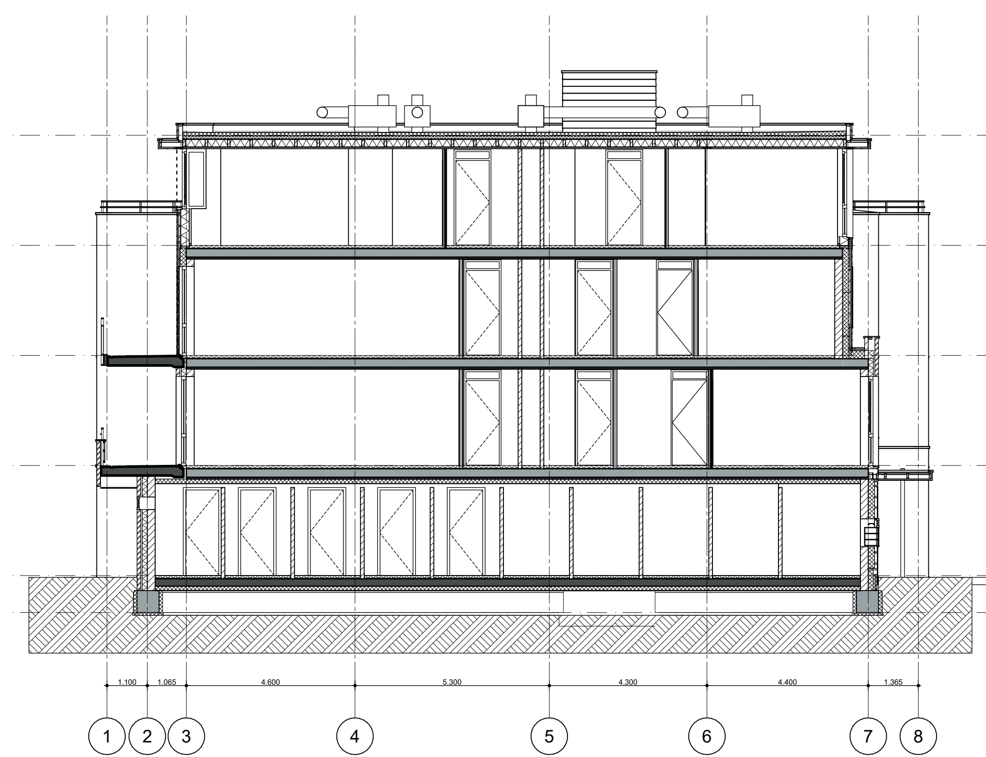
Doorsnede F-F
