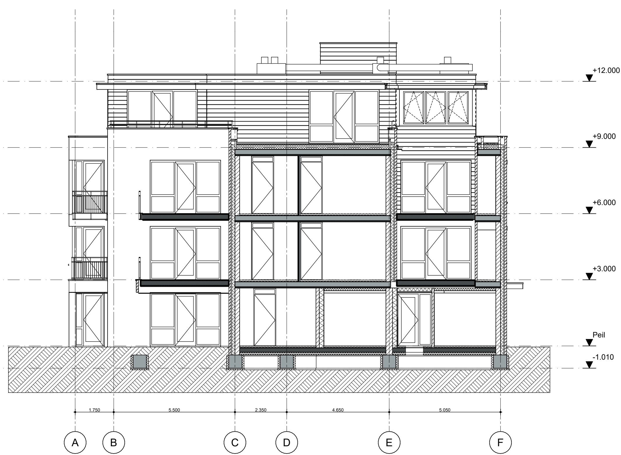
Doorsnede E-E
