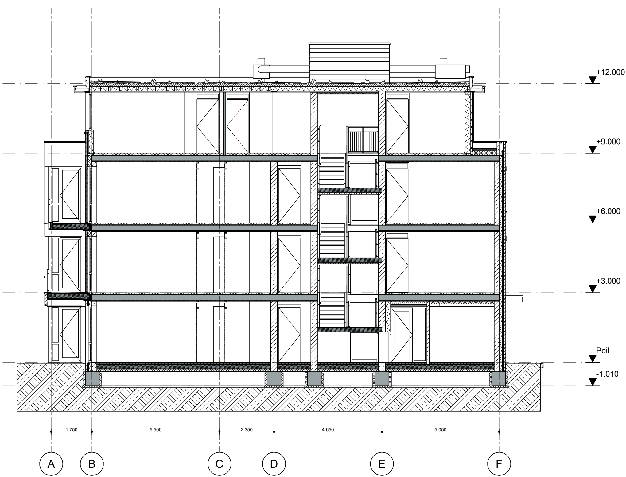
Doorsnede A-A
