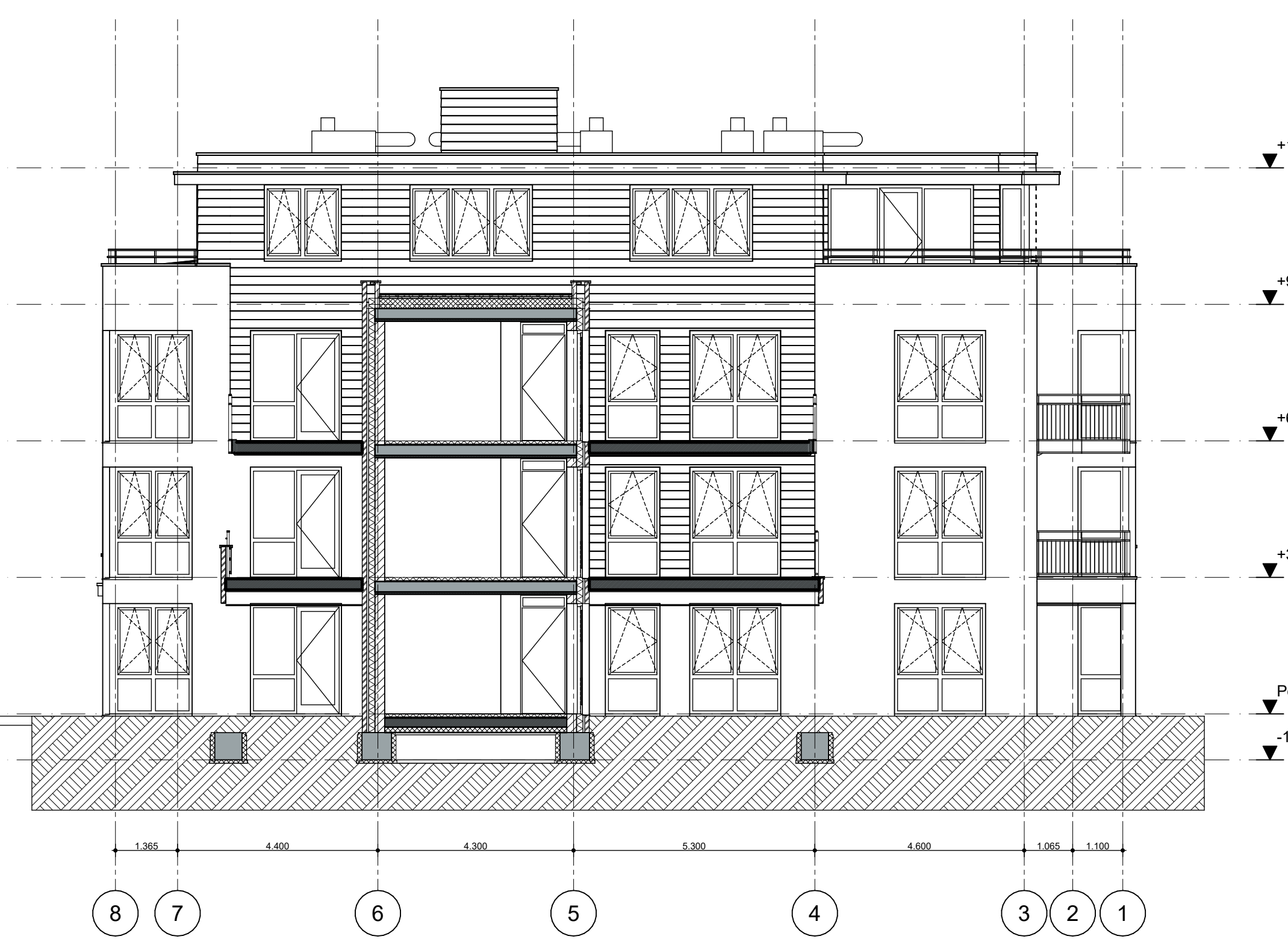
Doorsnede H-H
