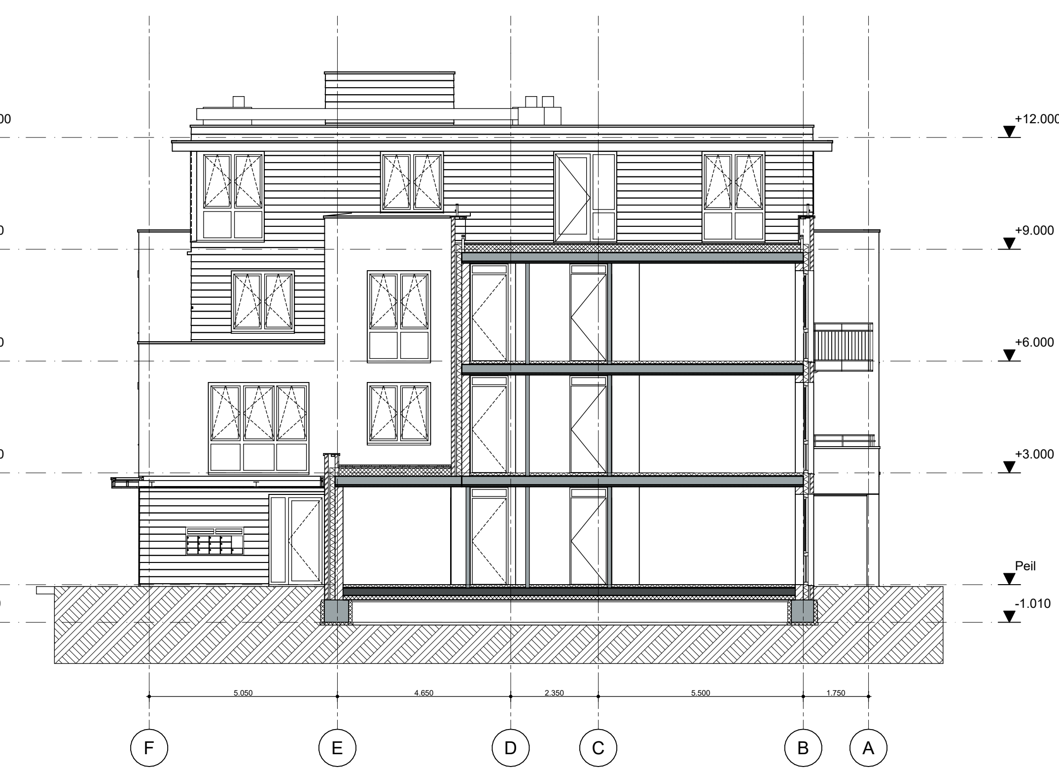
Doorsnede G-G
