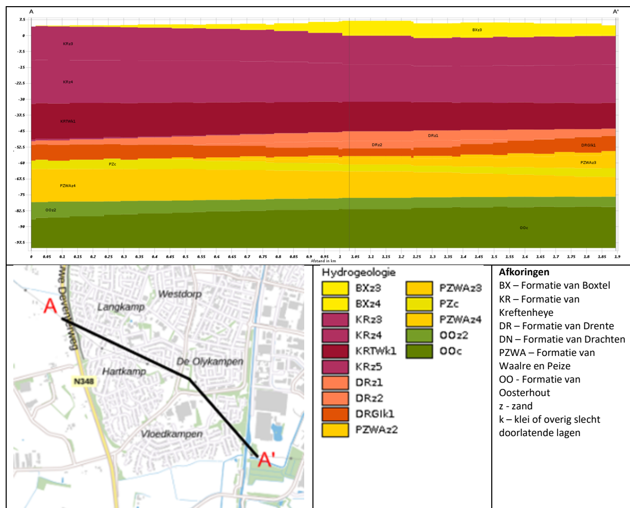
Figuur 3.1: Geohydrologische bodem structuur (bron: REGIS II.2, Dino-loket)
