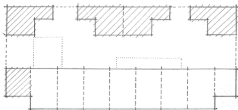
Transformatie van voormalige St. Jozefschool tot woningen in 2020 Slopen van een deel van de uitbreiding uit 1955 en het sanitaire blok uit 1993. Acht woningen in de voormalige school, waaronder een kangoeroe woning in de bestaande kop van de voormalige school. Daarnaast toegevoegd een kangoeroe woning in de nieuwe kop aan de andere zijde van de voormalige school en vier woningen aan de noordzijde, deze kunnen gekoppeld worden met de woningen in de voormalige school t.b.v. mantelzorg.
