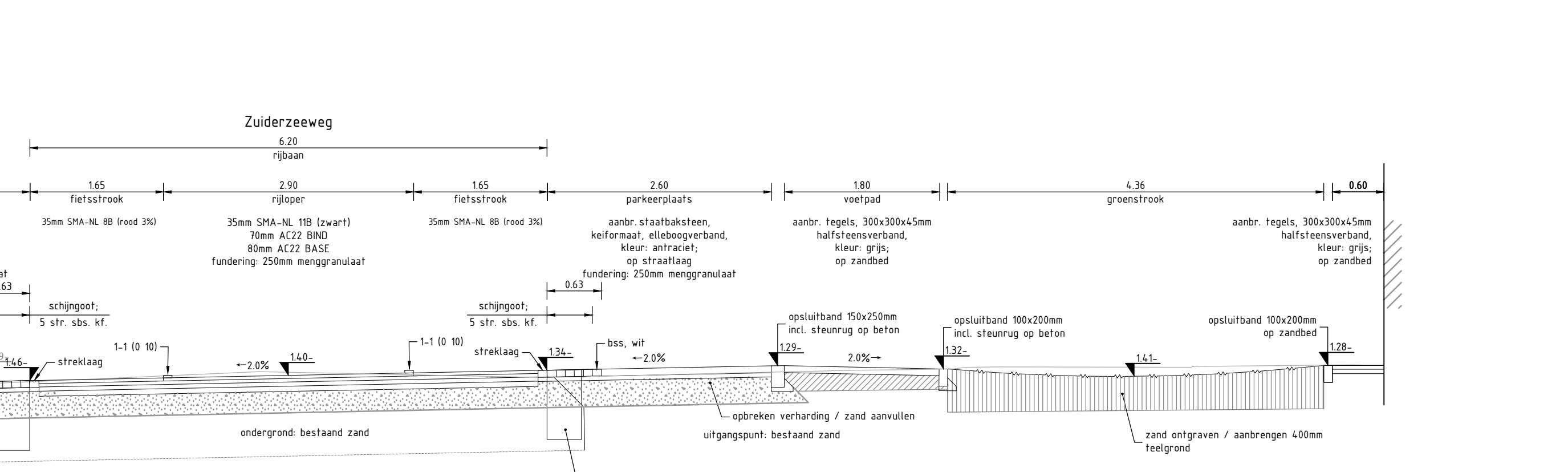
Detail Zuiderzeeweg schaal: 1 : 50
