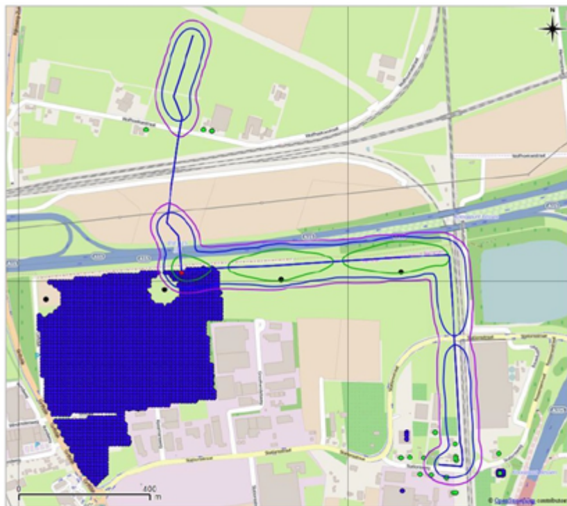
Figuur 3 Ligging van gastransportleiding N-578-19 (blauw). De locaties van de windturbines zijn weergegeven met zwarte stippen. De contouren van het PR van 10^{-6} , 10^{-7} en 10^{-8} per jaar van de leiding worden weergegeven met respectievelijk groen, blauw en paars.
