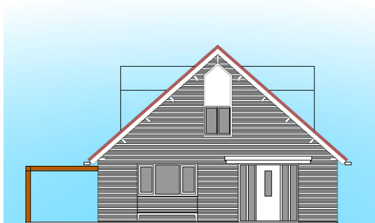
ZUIDGEVEL
