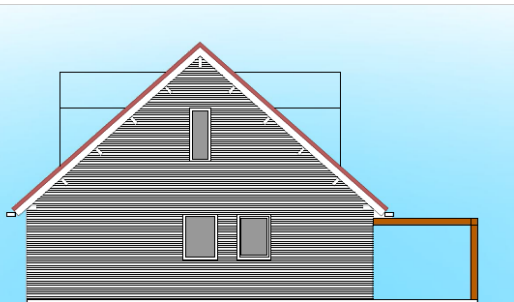
NOORDGEVEL
