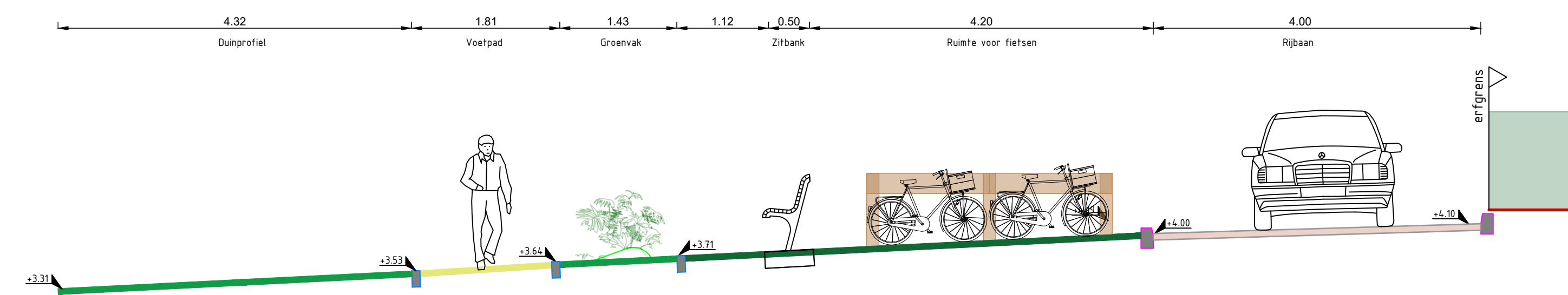
Dwarsdoorsnede 1-1 Groene Strand Schaal 1/50
