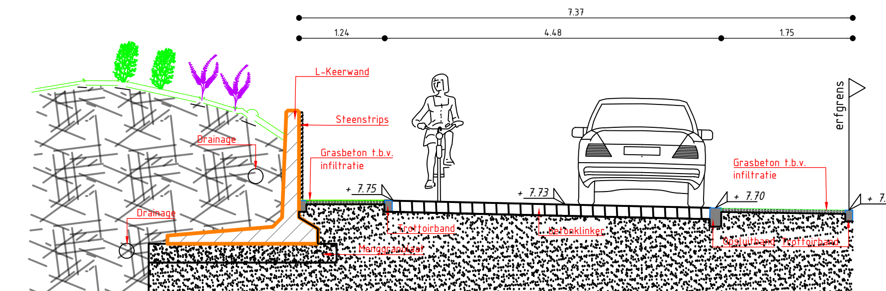
Dwarsdoorsnede A-A Zwarteweg Schaal 1/50
