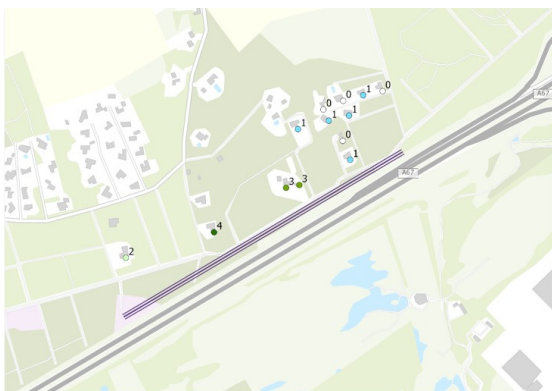
Geluidsreductie met wal van 4 meter hoog
