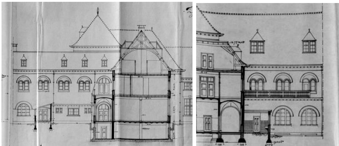
De geveltoestand op tekeningen uit 1922, beide gevels aan de zijde van de binnenplaats.
