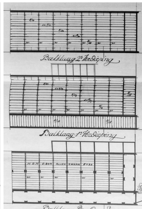
Doorsnede op tekening van april 1924. Rechts de vloerconstructies op tekening van dezelfde maand.
