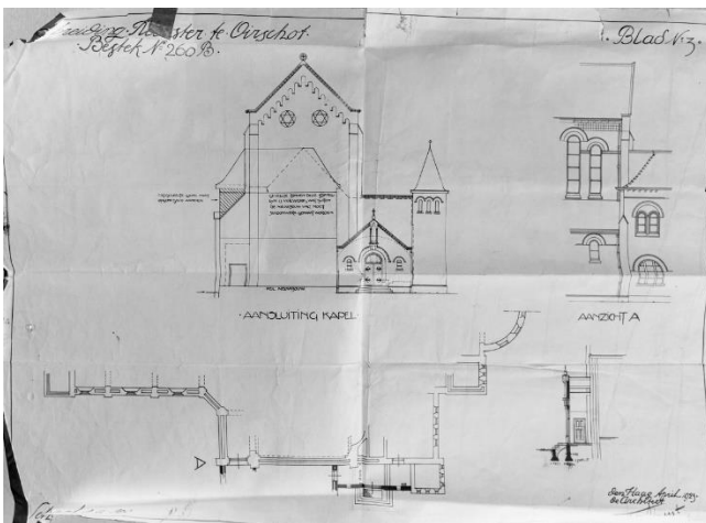
Het aangebouwde portaal uit 1923. Links bouwtekening, rechts thans bestaande toestand.
