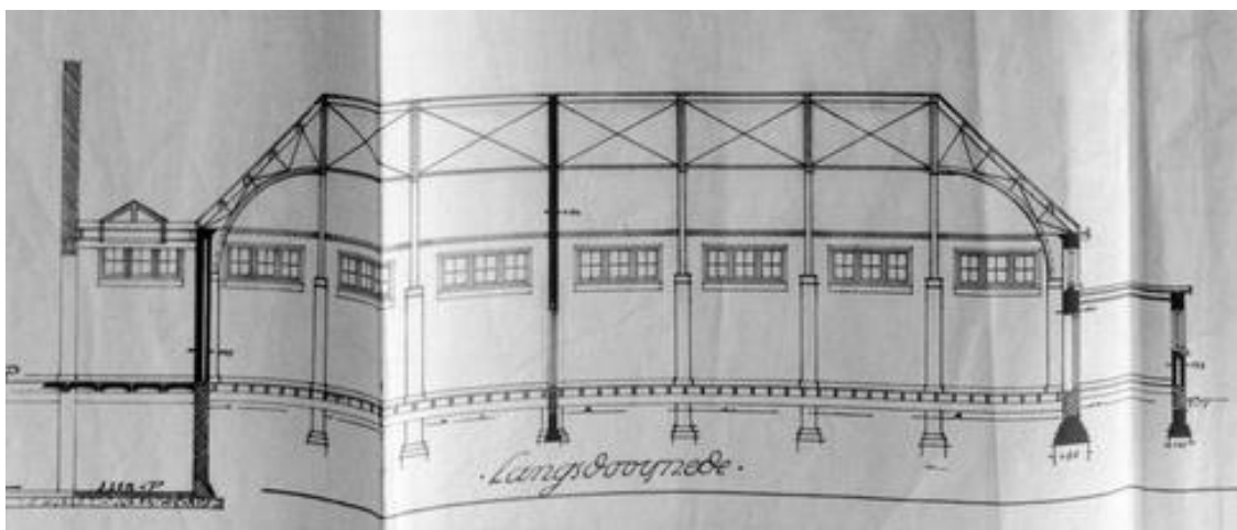
Doorsnedertekening waarop onder andere de in steel uit te voeren kapconstructie is te zien.
