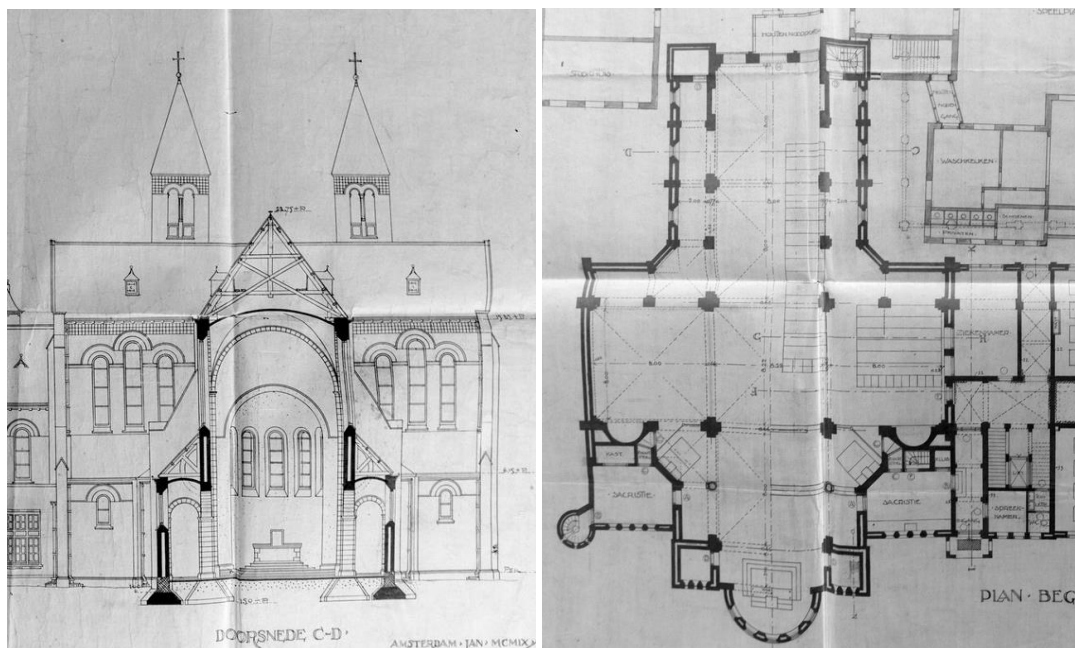
Detail bestek 173b bladnr 5. Detail bestek 173b bladnr 2. Doorsnede en plattegrond.
