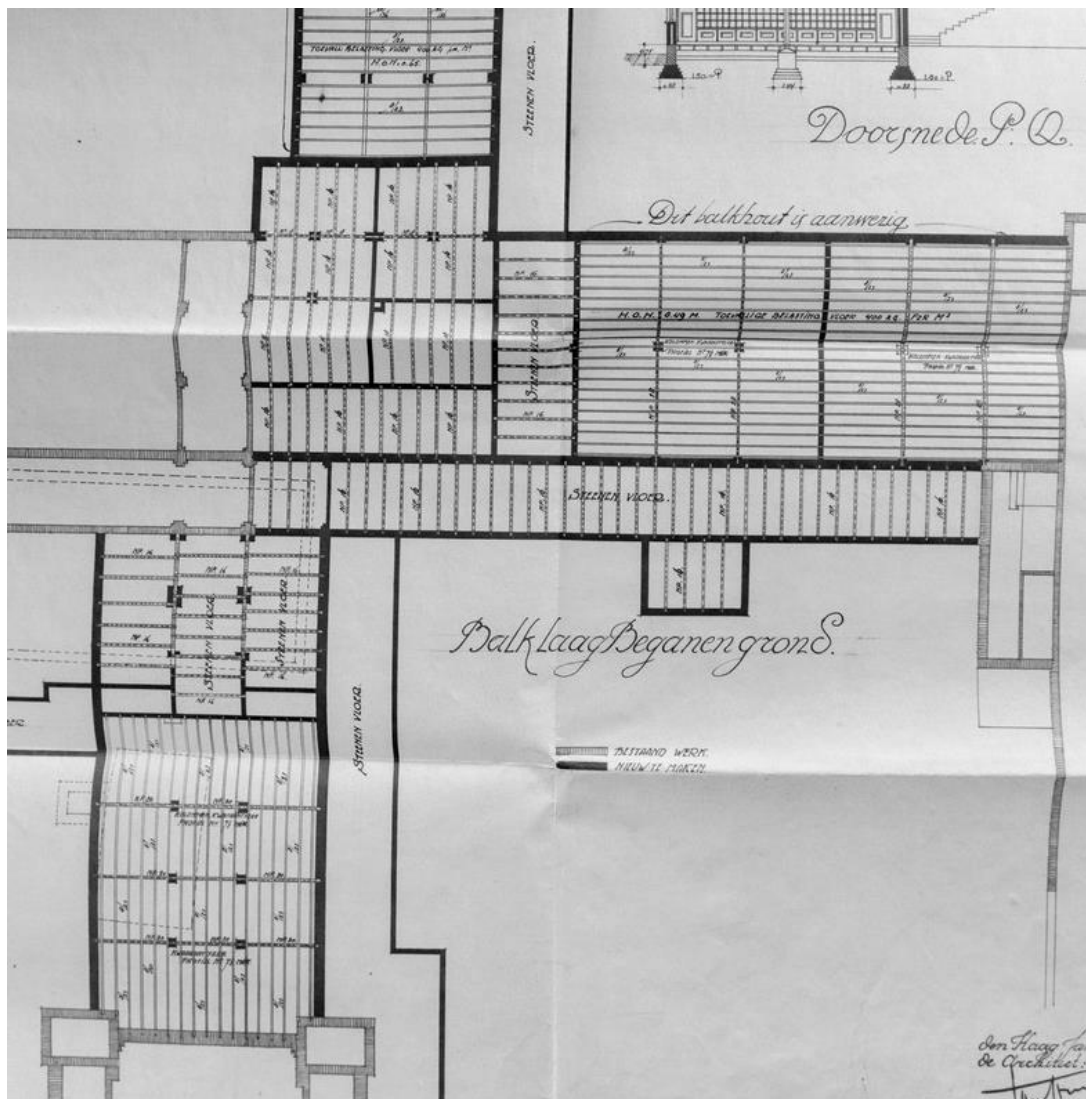
De balklaag van de begane grond op tekening van januari 1925 met deels stenen vloeren en deels houten vloeren (refter, recreatie en bidkapel).
