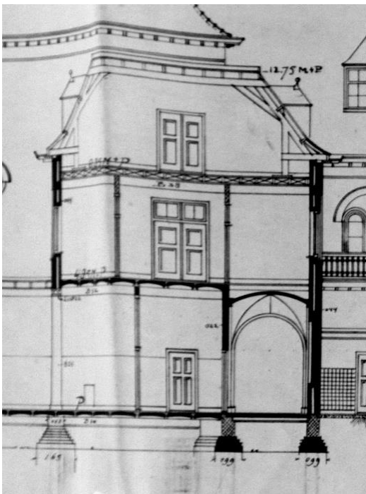
Detail van de constructie met gehakte merken II.
