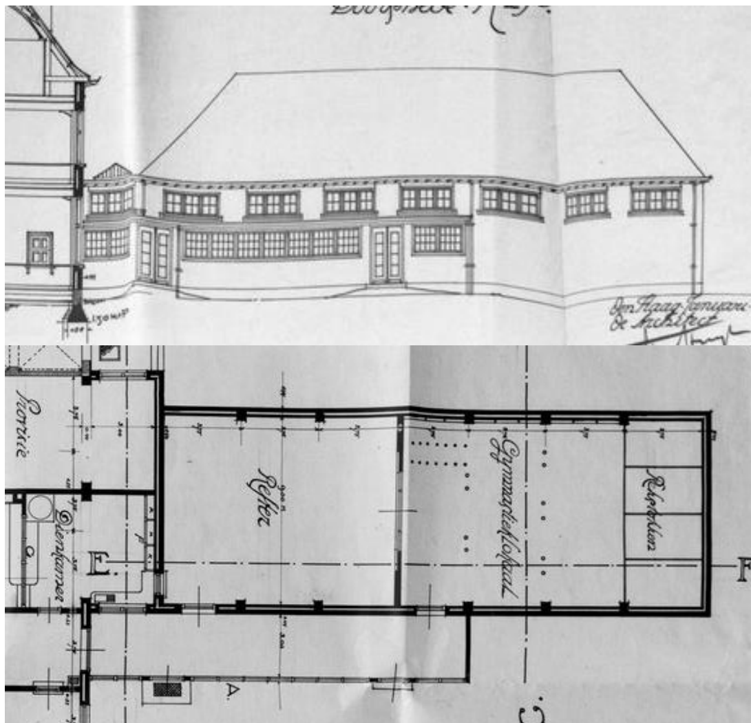
Combinatie van plattegrond- en geveltekeningen van januari 1925.
