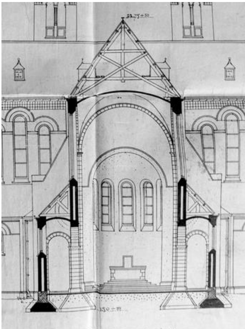
Detail van een tekening uit 1908 met doorsnede over het schip van de kapel. Spouwmuren, trasraam, gemetselde gewelven en de kapspanten zijn te zien.
