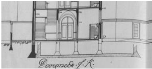
Doorsnedetekeningen uit 1925 met links de tongewelfde kelder onder het bidkoor (links) en de laatnegentiende-eeuwse kelder grotendeels onder de kloostergang (rechts), ontdaan van kelderdek.
