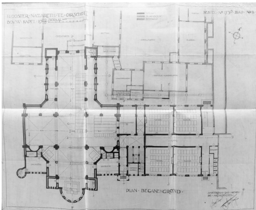
Vóór de Eerste Wereldoorlog werden de nieuwe Kweekschool én de nieuwe kapel gerealiseerd. Hier de nieuwe kapel in plattegrond.
