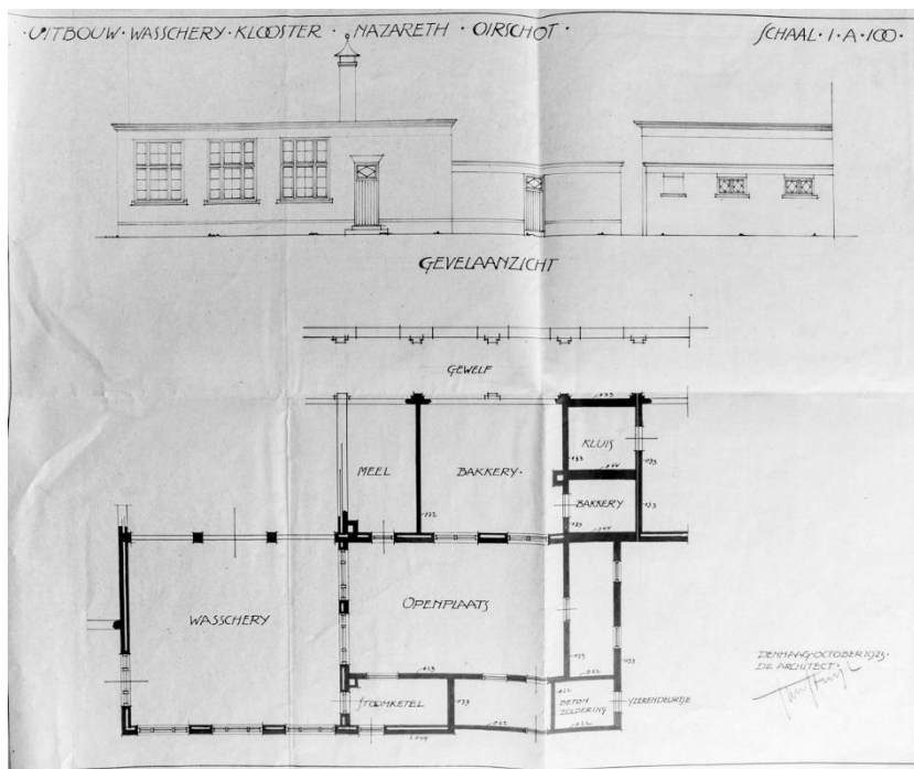
Bouwtekening van oktober 1923 met bakkerij, open plaats en ruimte voor de stoomketel.
