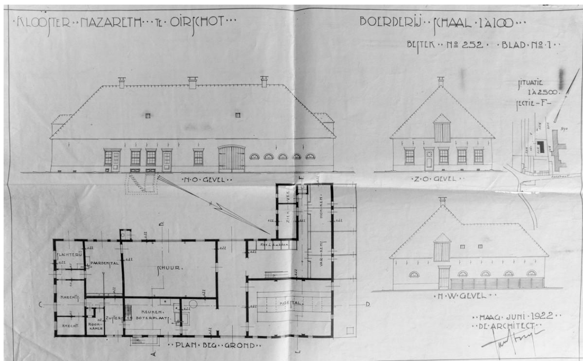
Bouwtekening voor de nieuwe boerderij, juni 1922.
