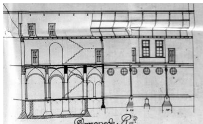
De doorsnedetekeningen die over de bidkapel gaan. Poeren onder kolommen zijn te zien, alsmede de gemetselde troggewelfjes, de gemetselde kruisgewelven in de gang en de houten balklaag van de zoldervloer. In de dwarsdoorsnede ook het principe van de kap.
