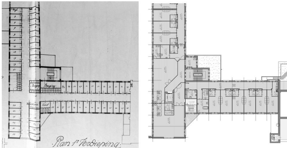
De tekening van de toestand in 1923 (links) wijkt compleet af van de thans bestaande toestand. Van de middengangen, de cellen en de bergingen is niets meer over.
