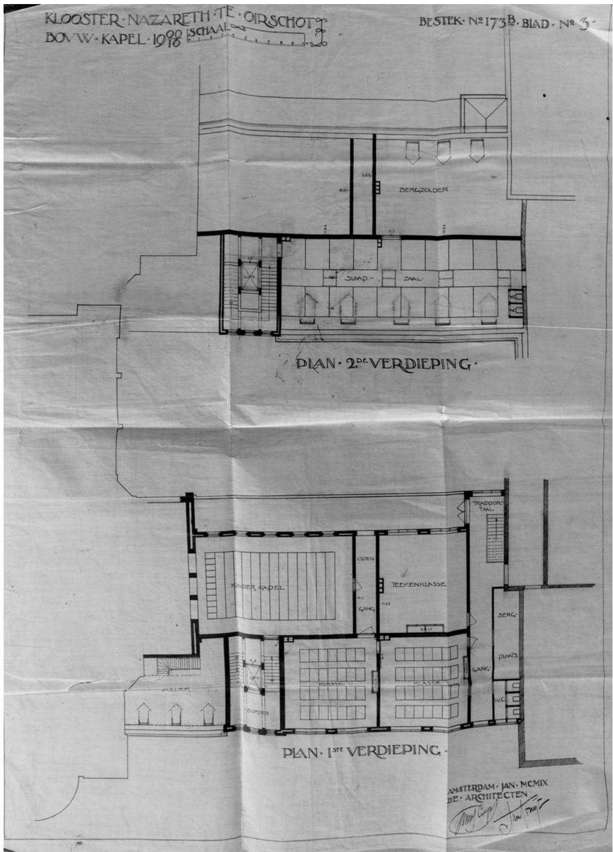
Detail bestek 173b bladnr 3. De kapel op de verdieping was als kinderkapel bedoeld, zo blijkt uit tekening van Cuypers en Stuyt.
