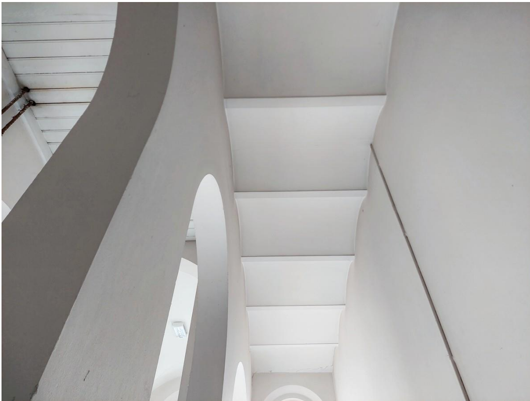
De zoldervloer van het trappenhuis bestaat uit troggewelfjes tussen stalen liggers. Linksboven op foto het liftgat.
