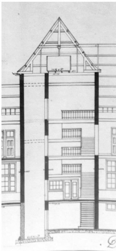
Detail van de constructietekening uit 1922 (let op het waterreservoir) en de thans bestaande toestand met op de voorgrond de stalen balk waarop het reservoir rustte.
