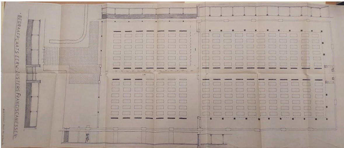
Tekening uit 1962 met een plan voor uitbreiding van de begraafplaats. Vermoedelijk kwamen pas na die tijd de eerste grafkruizen op de begraafplaats.
