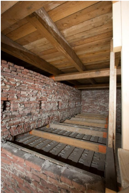
Deel van het platte dak van de sacristie (boven de kasten van de voormalige gerfkamer). Rechts de met hout omklede stalen balk van het zangkoor.
