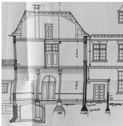
De doorsnedetekeningen die over de bidkapel gaan. Poeren onder kolommen zijn te zien, alsmede de gemetselde troggewelfjes, de gemetselde kruisgewelven in de gang en de houten balklaag van de zoldervloer. In de dwarsdoorsnede ook het principe van de kap.
