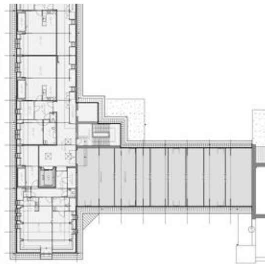
De zolder op tekening uit 1923 (links) en de tekening van de thans bestaande toestand. Transformatie heeft in de zijvleugel plaatsgevonden.
