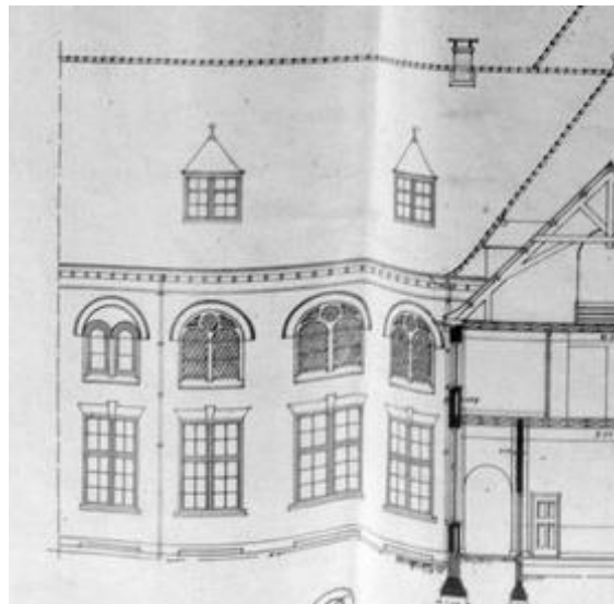
De gevel aan de zijde van de achtertuin. Rechts de toestand op tekening uit 1922, zonder aanbouw en met oratoriumvenster op de verdieping. Dakkapellen hebben plaatsgemaakt voor een dakterras en dakramen.
