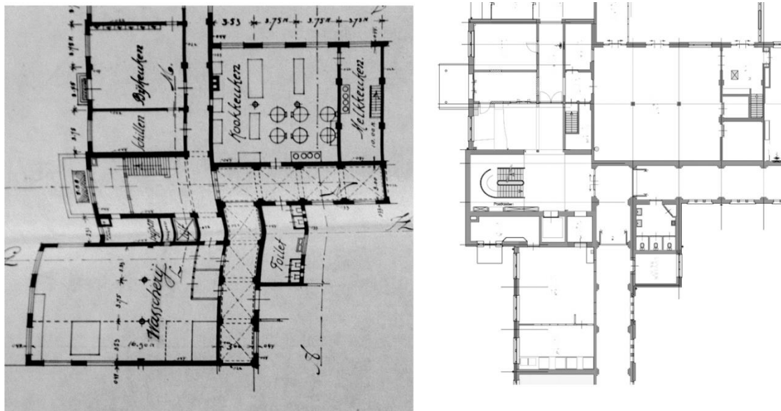
De vergelijking van de tekening uit 1922 met de huidige toestand, laat grote verschillen zien, doch ook constanten op het niveau van de hoofdstructuur (met name kloostergang en keuken).
