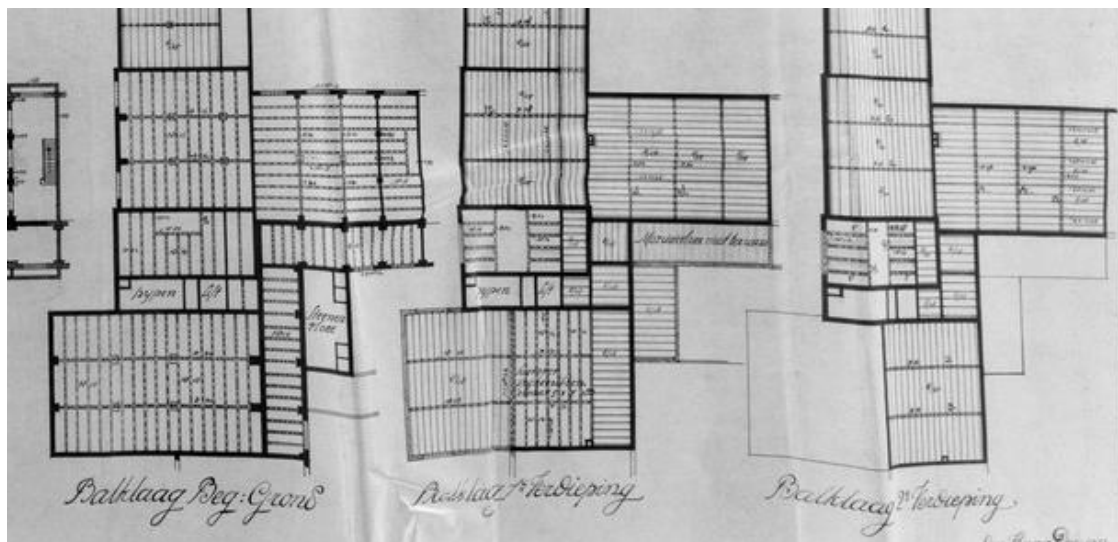
Detail van de constructietekening uit 1922 met vloeren van de begane grond en de verdiepingen.
