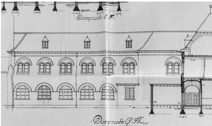
De gevel aan de kloosterhof in op de ontwerptekening.
