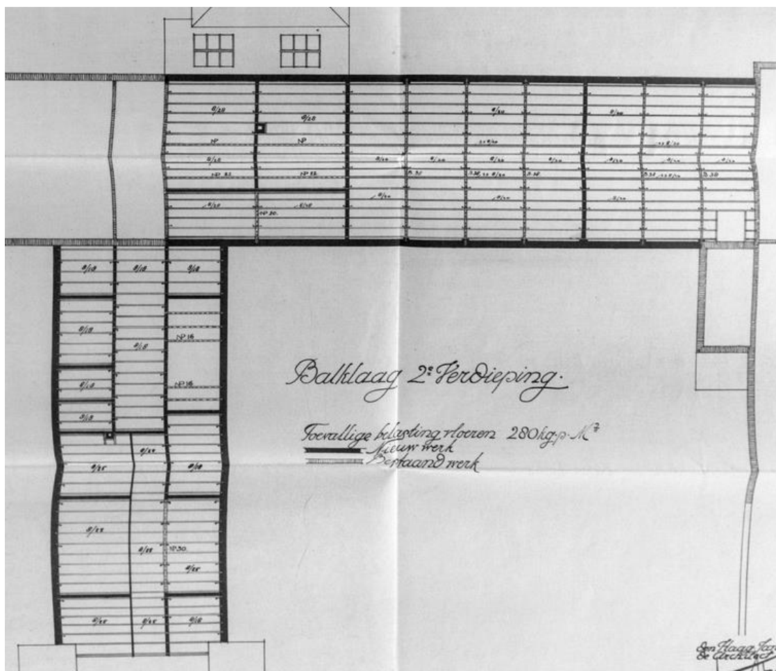
De vloerconstructie van de balklaag van de zolder.
