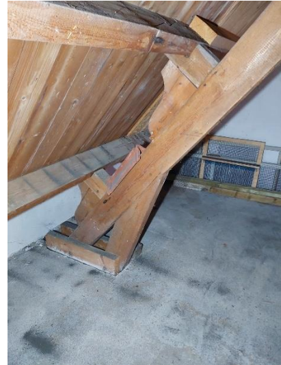
De toevoeging van een verdiepingsvloer in de vroegere kapel van de kweekschool heeft geresulteerd in toevoeging van constructies en aanpassing van bestaande (rechts zijn spantbeen en kreupele stijl bijvoorbeeld ingekort).
