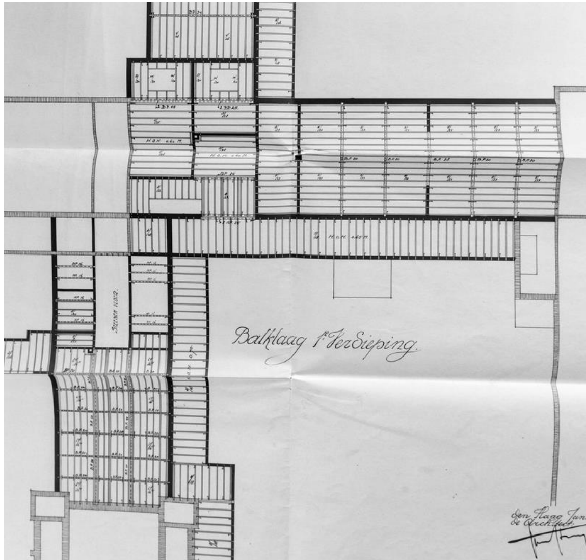
De tekening van de vloerconstructie van de eerste verdieping.
