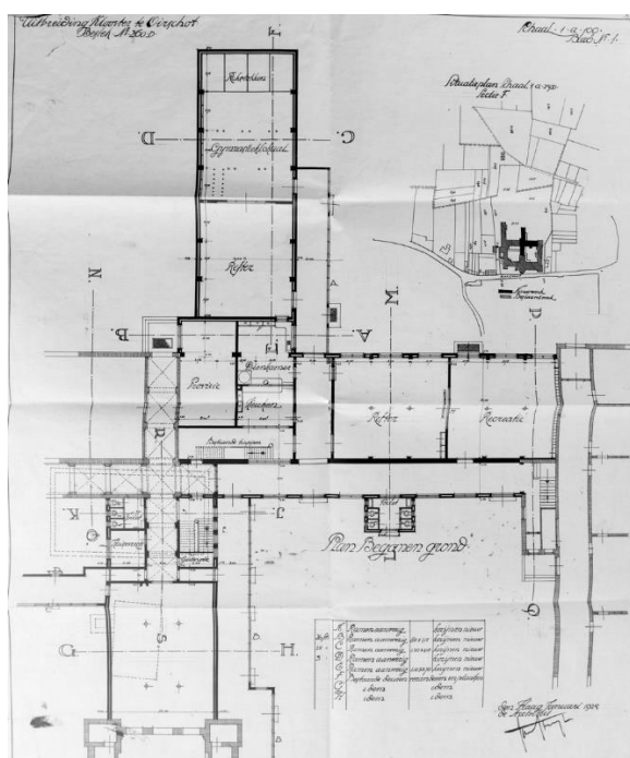
De plattegrond van de begane grond, bestektekening januari 1925 met rechts de thans bestaande toestand.
