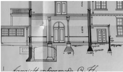
Doorsnedetekeningen uit 1925 met links de tongewelfde kelder onder het bidkoor (links) en de laatnegentiende-eeuwse kelder grotendeels onder de kloostergang (rechts), ontdaan van kelderdek.
