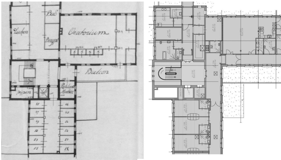
De verdieping op tekening uit 1922 links naast de huidige toestand. Herinnering aan de begintijd zijn vrijwel geheel verdwenen. Kolommen zijn behouden gebleven. Wellicht zijn er nog oudere afwerkingen achter latere toplagen weggewerkt.
