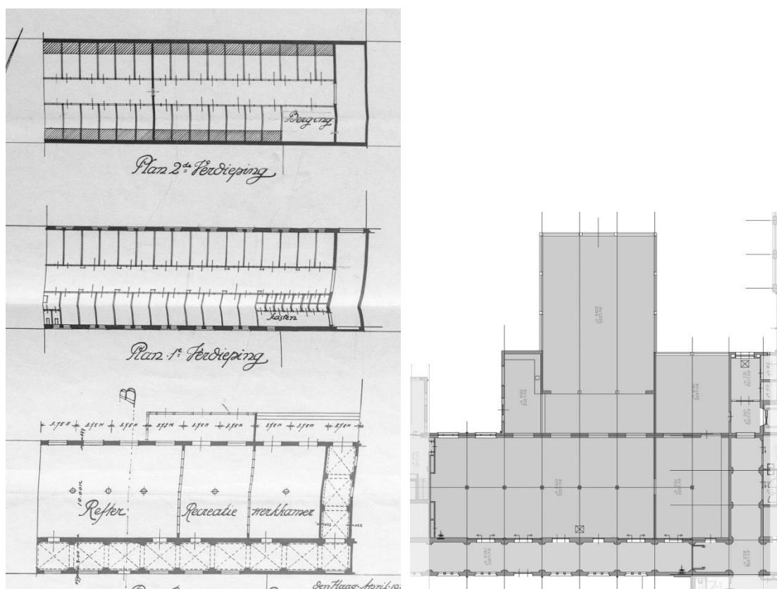
Bestektekening van april 1924 (links) en de huidige plattegrond van de begane grond.
