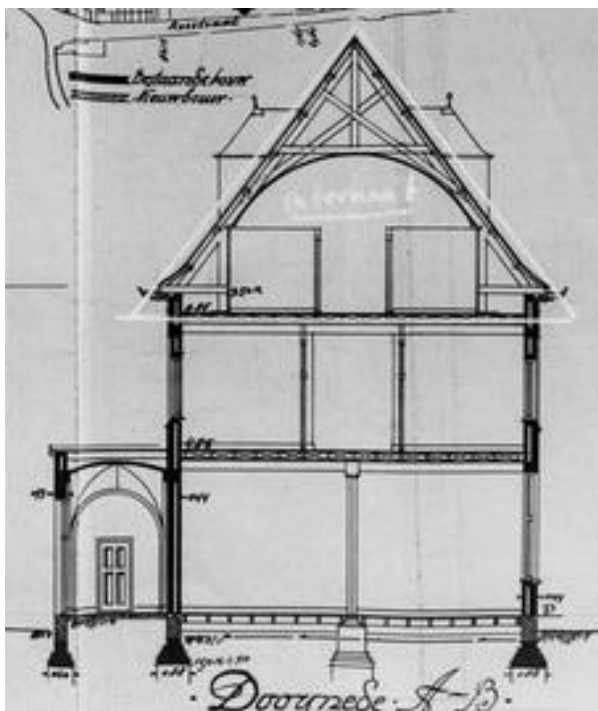
Doorsnede op tekening van april 1924. Rechts de vloerconstructies op tekening van dezelfde maand.
