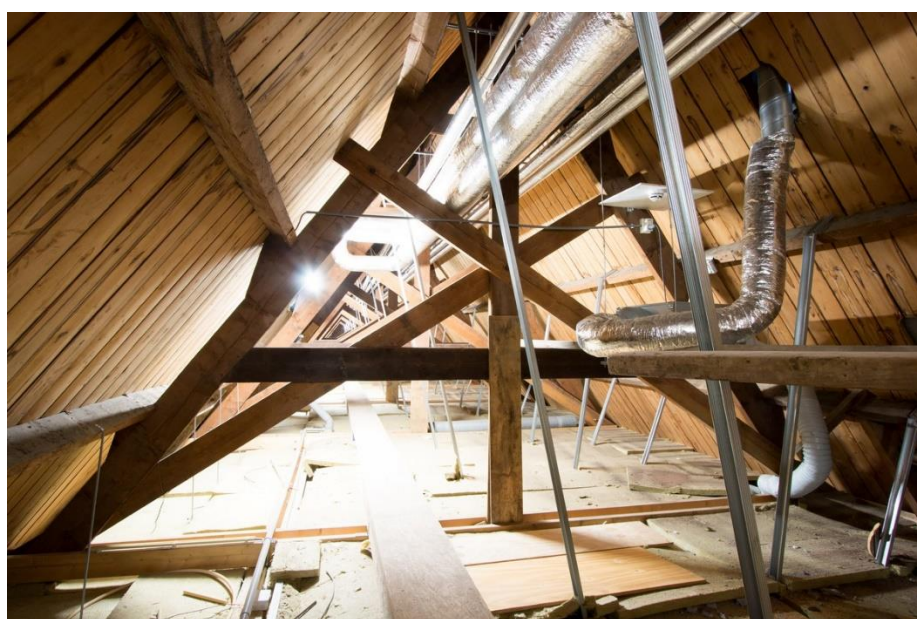
Deel van de spanten boven de secundaire plafonds. Hier is het tongewelf geheel verdwenen.
