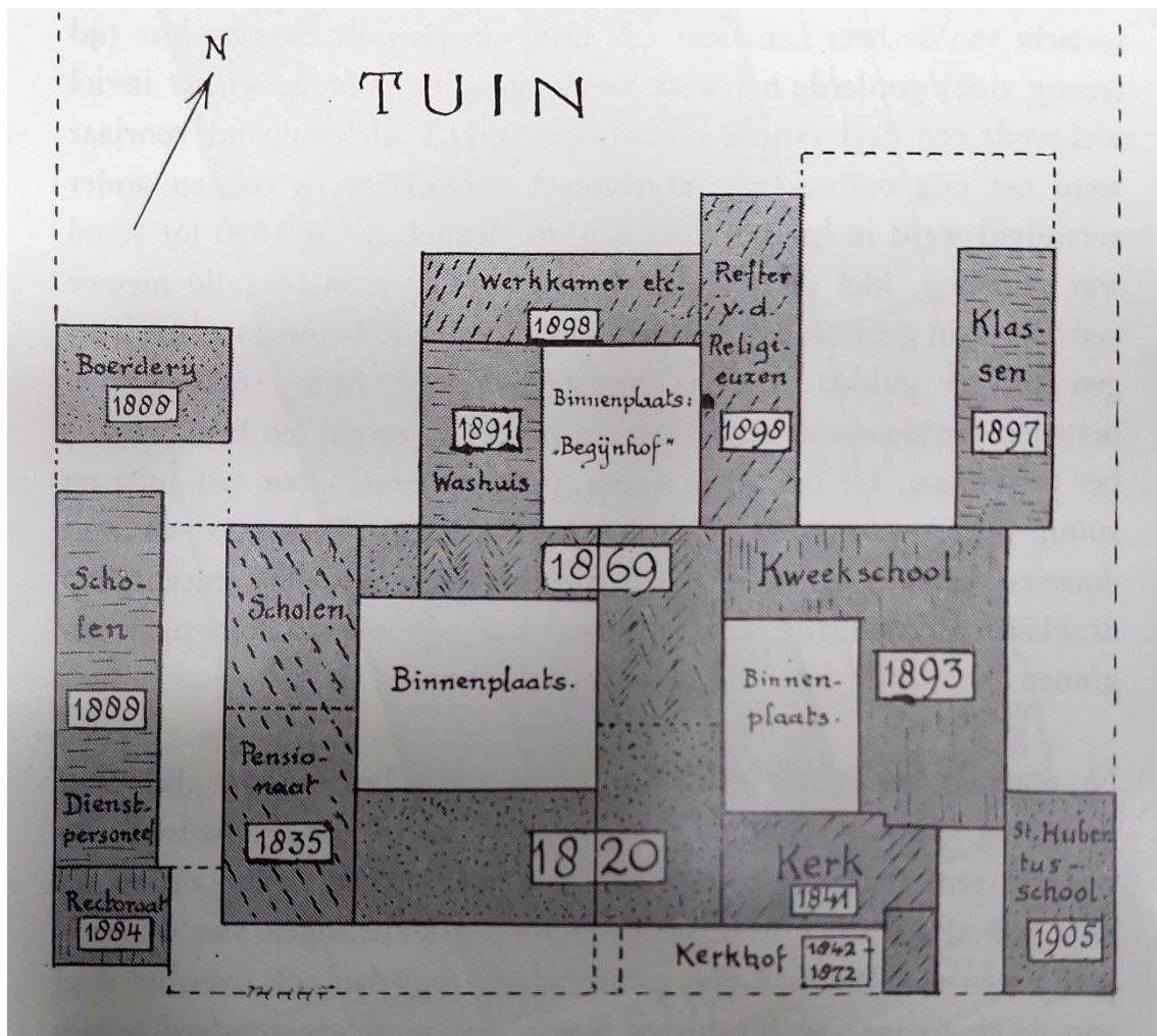
De schetsmatige weergave van het complex op het moment dat Cuypers en Stuyt een nieuw masterplan maakten. Sommige te slopen gebouwen waren op dat moment nog geen tien jaar oud. De tekening toont ook de plaats van de eerste kerkhof van het klooster, in gebruik tussen 1842 en 1872.
