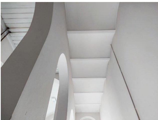
Verdiepingvloeren bestaan uit stalen liggers met daartussen gemetselde troggewelfjes uit de bouwtijd.
