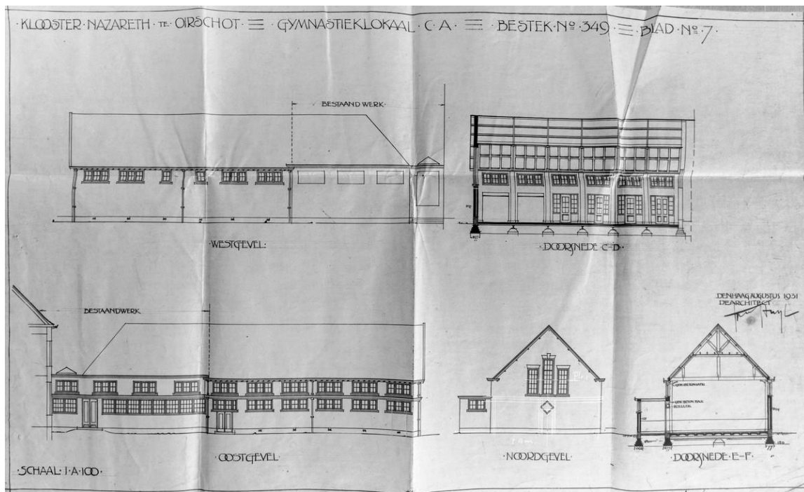
Tekening van de aanbouw van het gymnastieklokaal tegen de vijf jaar daarvoor gerealiseerde refter. Tekening augustus 1931.
