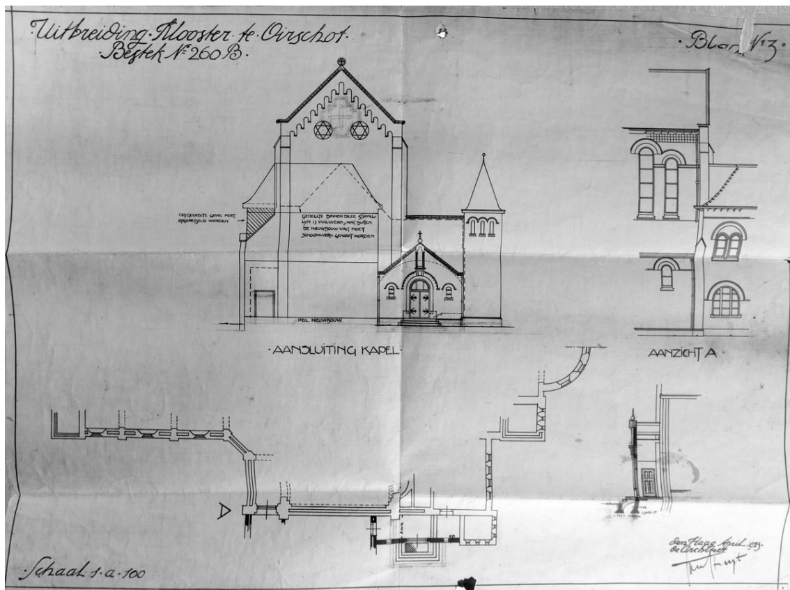
Detail bestek 260b bladnr 3. Aanbouw van een portaal naar plan uit 1923.
