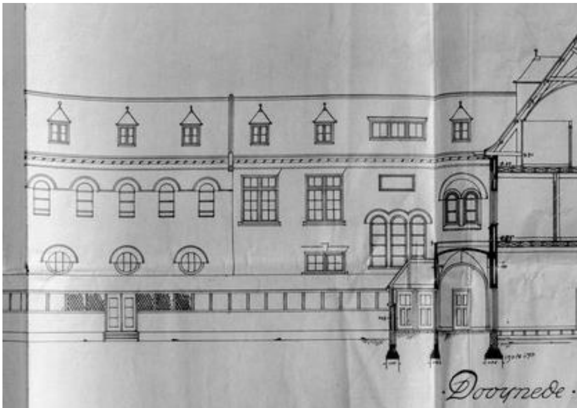
Ongedateerde bouwtekening die aan de tekening van januari 1925 vooraf moet zijn gegaan
