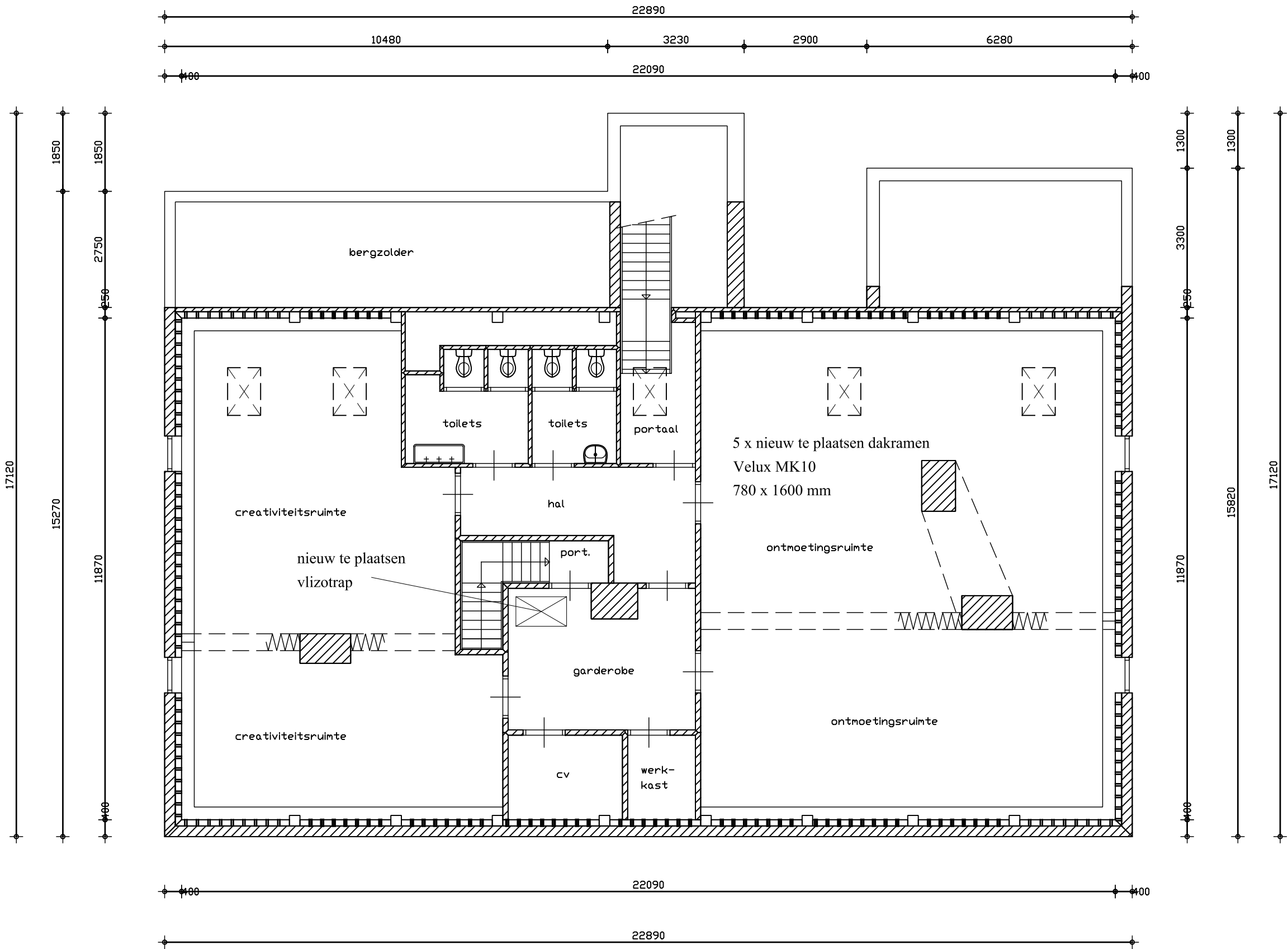
verdieping
