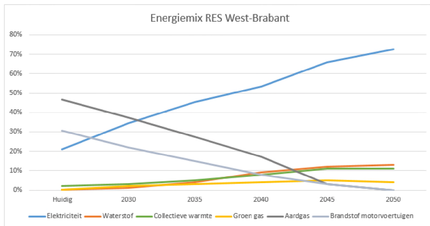
Figuur 1: Energimix West-Brabant
