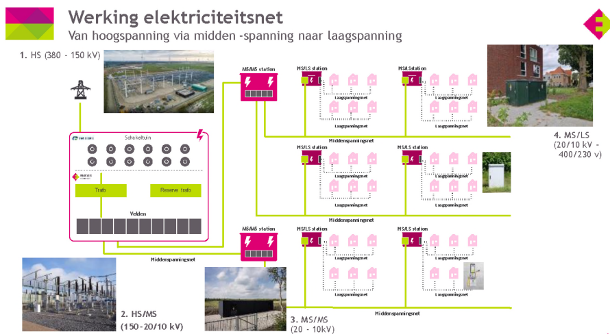
Figuur 6: Werking elektriciteitsnet
