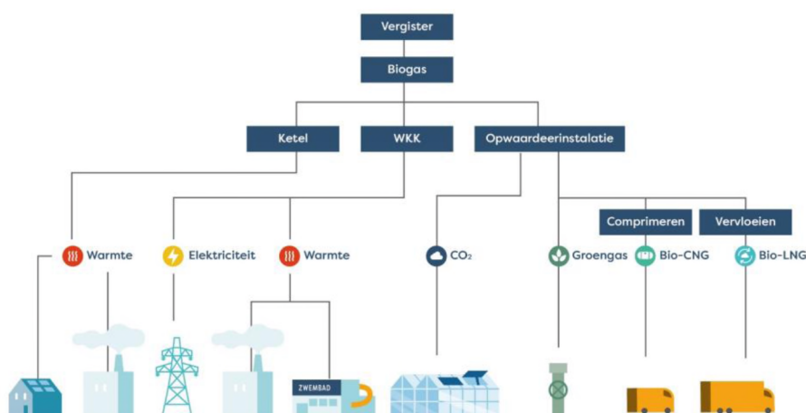
Figuur 9: Toepassingsmogelijkheden voor biogas, waaronder groen gasproductie
