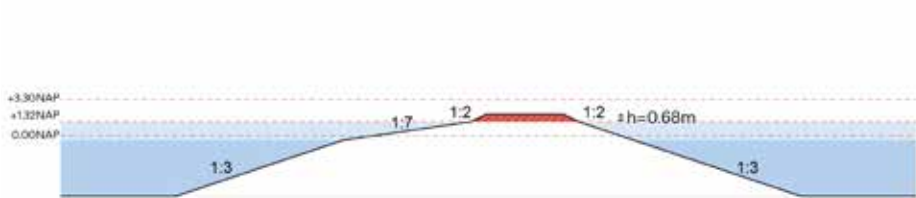
Langsdam B, C en EvB (+3.00 NAP)
