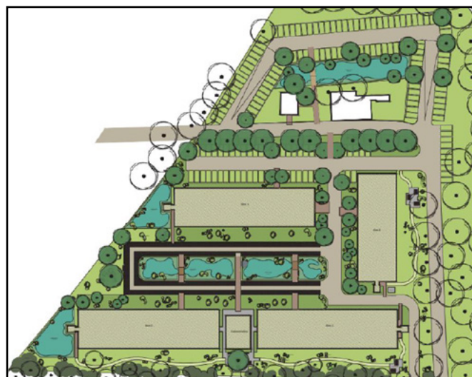
Situatietekening ingediende aanvraag omgevingsvergunning voor de huisvesting van 450 arbeidsmigranten aan de Blokdijk 1 in Moerdijk
