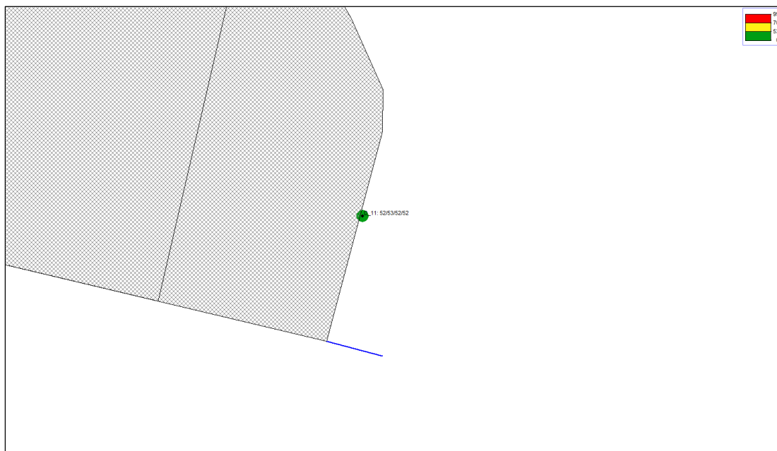
Figuur 5.1 Geluidluwe gevel door afschermende maatregel
