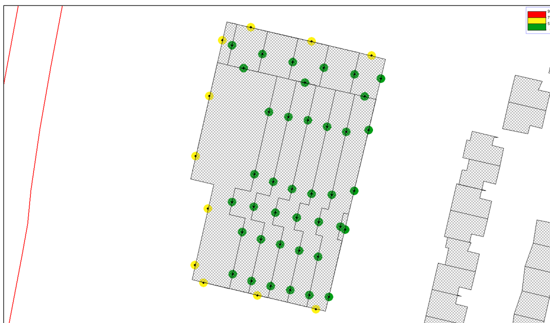
Figuur 4.3 Geluid door gemeentewegen op gevels bouwdeel C
