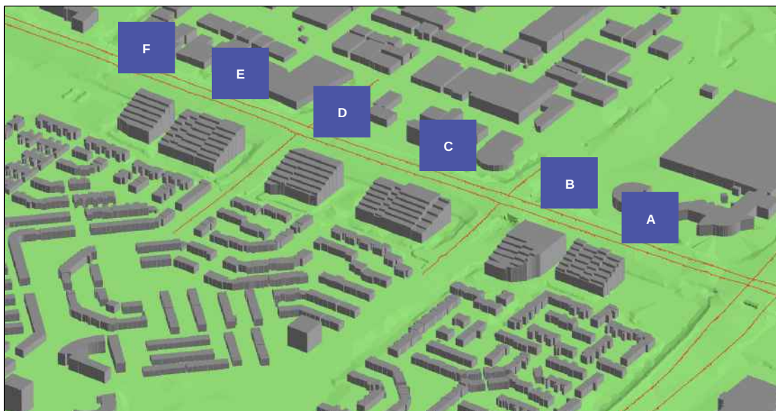
Figuur 3.1 3D-impressie rekenmodel inclusief benoeming bouwdelen
