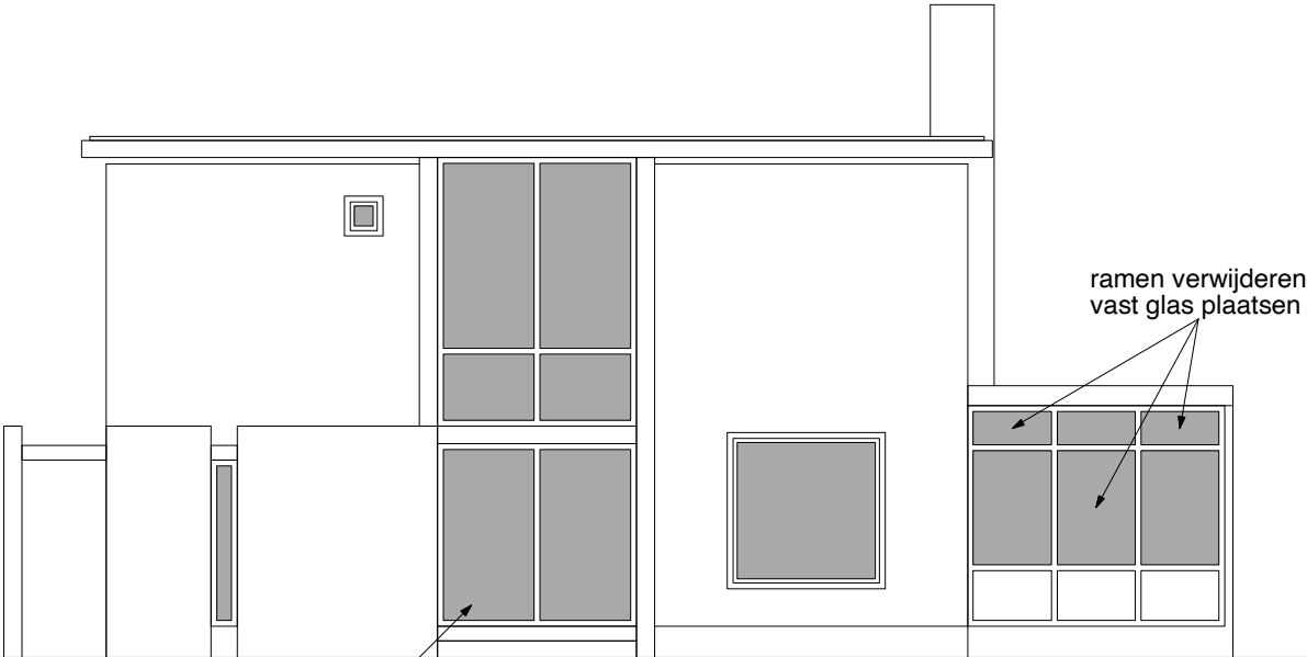
VOORGEVEL
