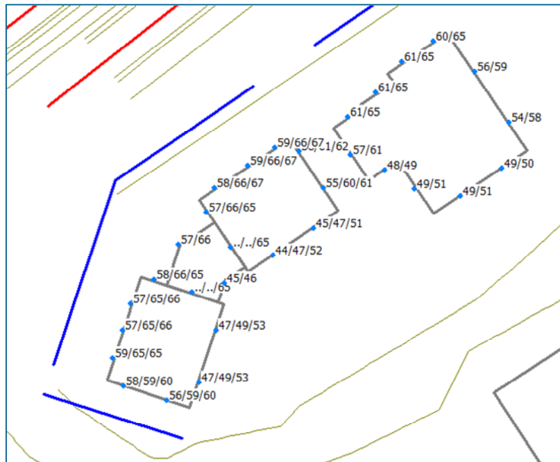
Afbeelding 4.3 Weergave geluidbelasting afkomstig van de N65 met scherm.
