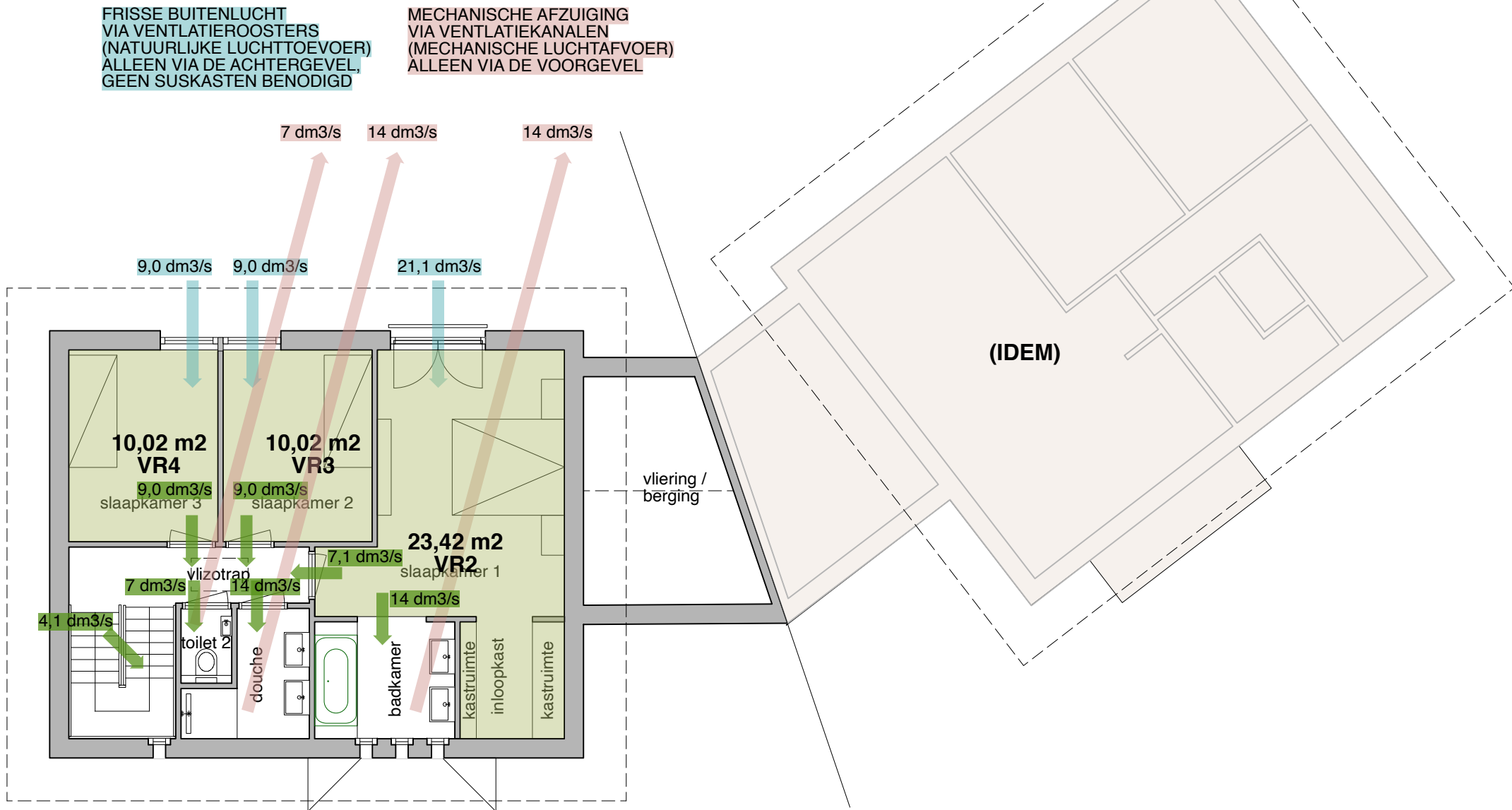
PLATTEGROND EERSTE VERDIEPING
