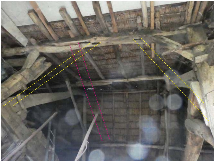
Gebintplaat tussen gebintstijlen C6 en C7. In geel de oude plaatsen van de schoren. In roze de vermoedelijk oude plaats van de eindplaat van het oorspronkelijke houtskelet.
