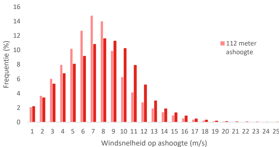
Figuur 29 Windsnelheidsverdeling op ashoogte voor een windturbine volgens de onder- (112 meter ashoogte) en bovengrens (140 meter ashoogte) van de onderzochte bandbreedte
