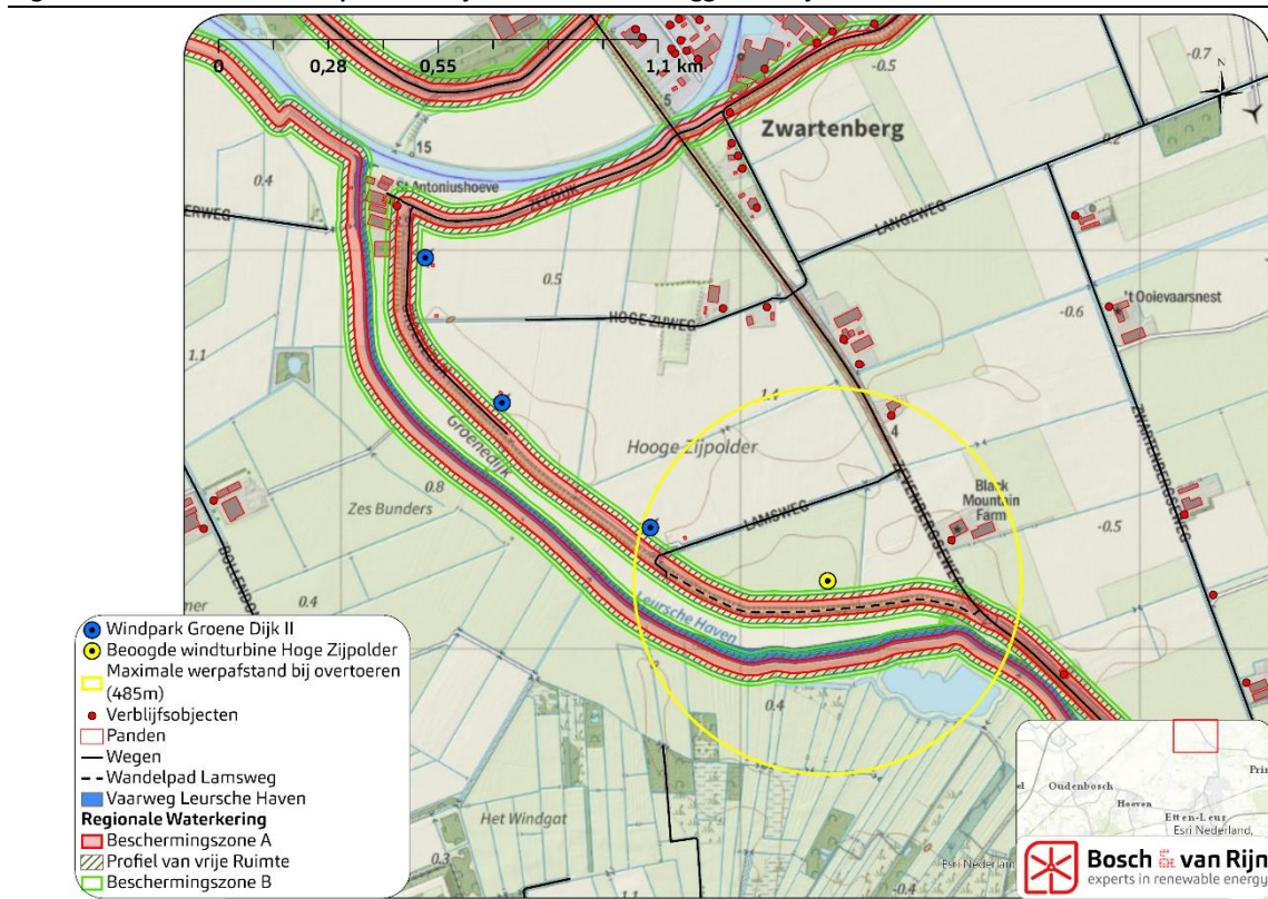
Figuur 11 Maximale werpafstand bij overtoeren en omliggende objecten.
