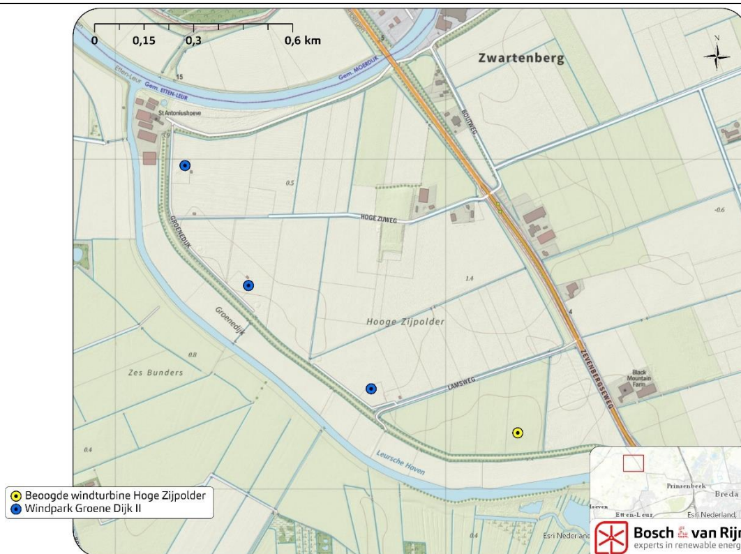
Figuur 17 Het beoogde initiatief de realisatie van windturbine Hoge Zijpolder (uitbreiding van windpark Groene Dijk II). Te zien is hoe de extra windturbine Hoge Zijpolder landschappelijk gezien in dezelfde lijnopstelling wordt gesitueerd.
