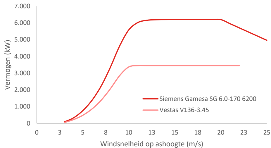
Figuur 30 Vermogenscurve voor een Vestas V136-3.45 windturbine en een Siemens Gamesa SG 6.0-170 6200 windturbine (gangbaar voor respectievelijk de onder- en bovengrens van de onderzochte bandbreedte)
