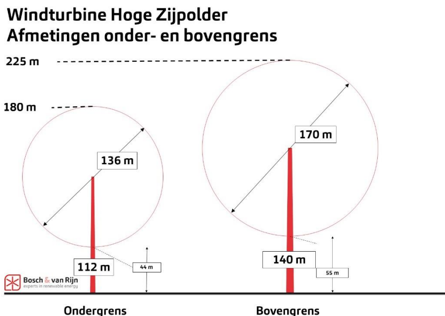
Figuur 3 Schematische weergave van de bandbreedte uit de vergunningaanvraag
