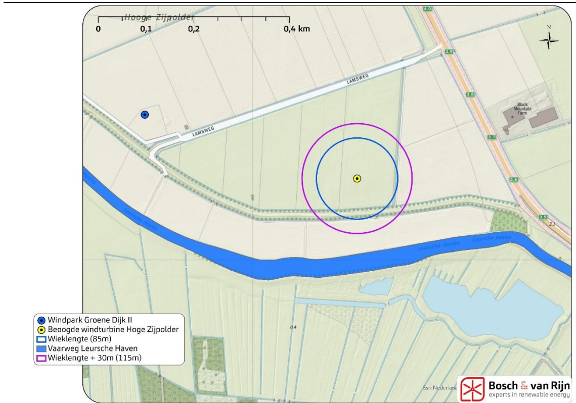
Figuur 14 Ligging van de vaarweg ten opzichte van de windturbine
