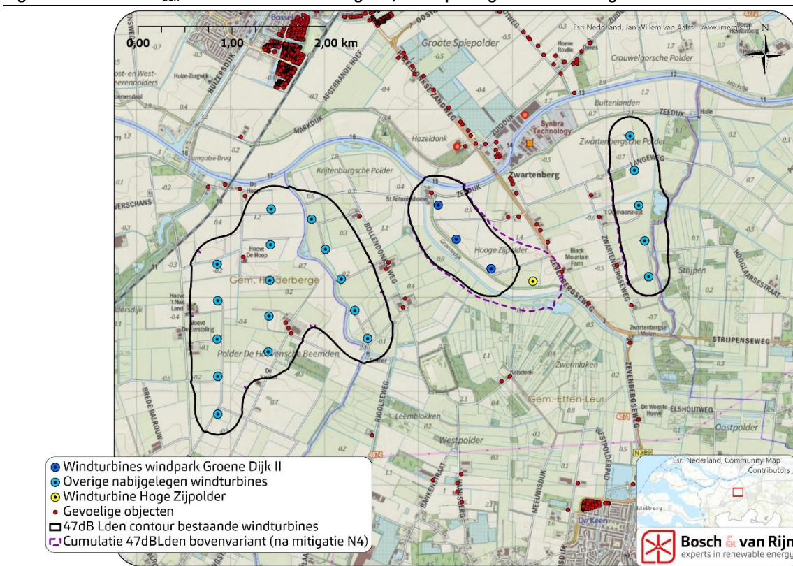
Figuur 7 47 dB L den -contouren van de bovengrens, na toepassing noise mode N4 gedurende de nacht
