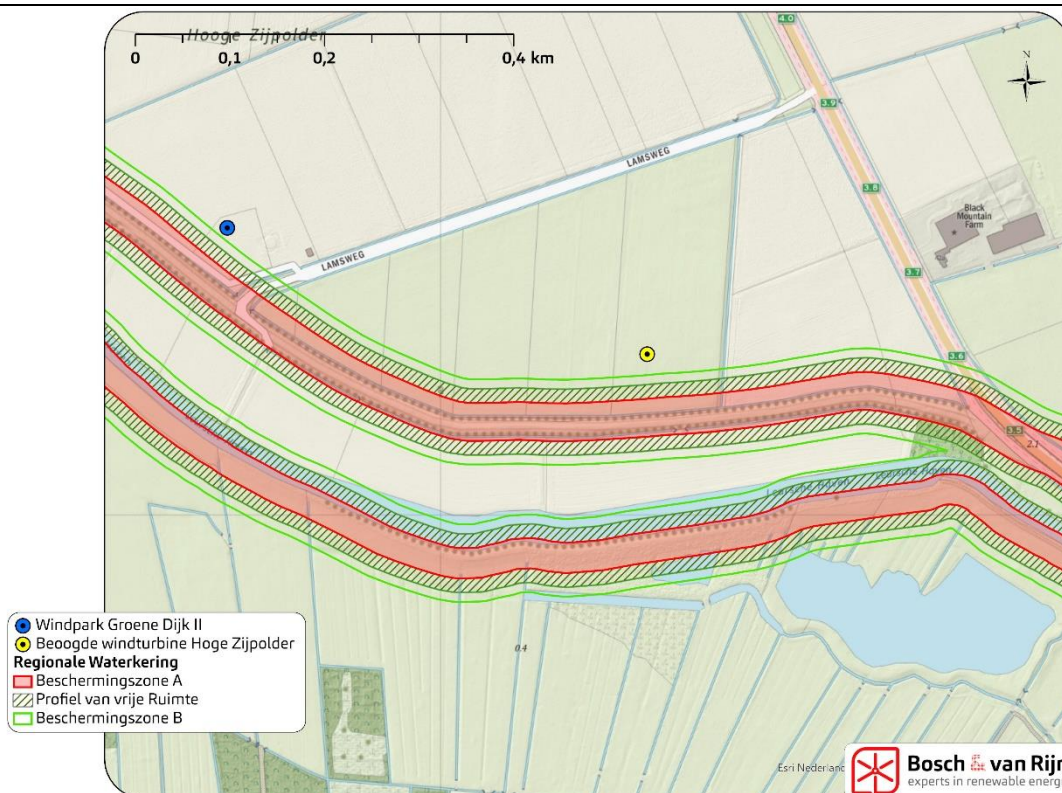
Figuur 15 Ligging van de waterkering ten opzichte van de windturbine
