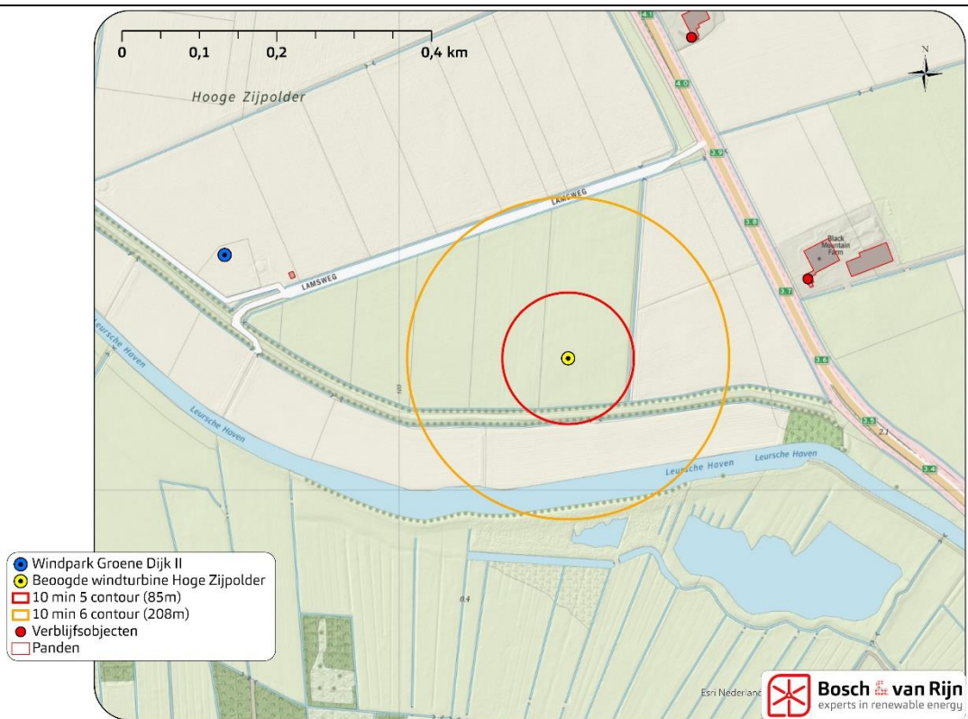
Figuur 12 Risicocontouren en (geprojecteerd) kwetsbare of beperkt kwetsbare objecten rondom de windturbine
