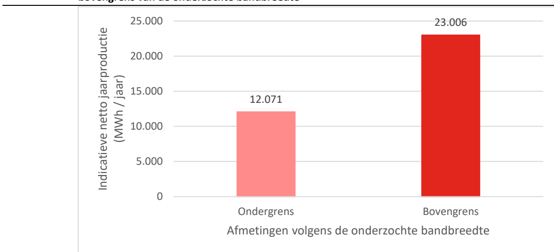
Figuur 31 Indicatieve opbrengst van de windturbine Hoge Zijpolder in geval van respectievelijk de onder- en bovengrens van de onderzochte bandbreedte
