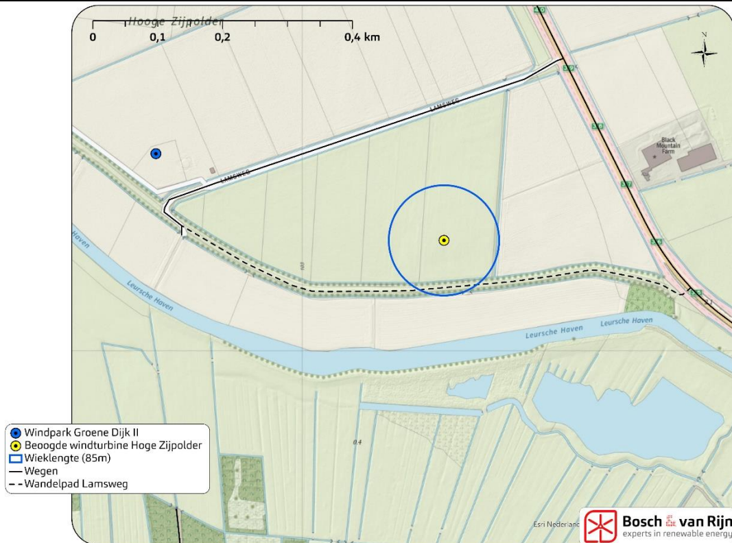
Figuur 13 Overdraai door de windturbine boven openbare wegen
