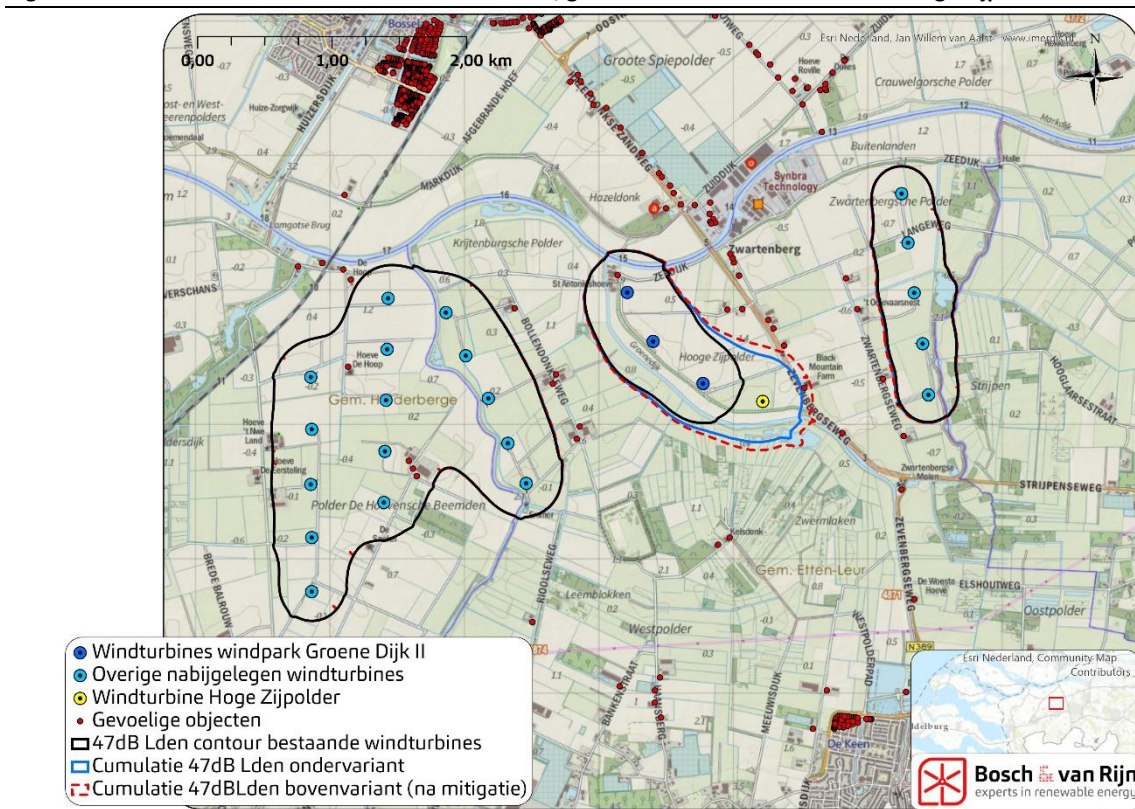
Figuur 6 Contouren van bestaande windturbines, gecumuleerd met de windturbine Hoge Zijpolder
