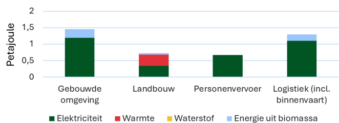
Figuur 10: vraag naar energie in de 0-variant
