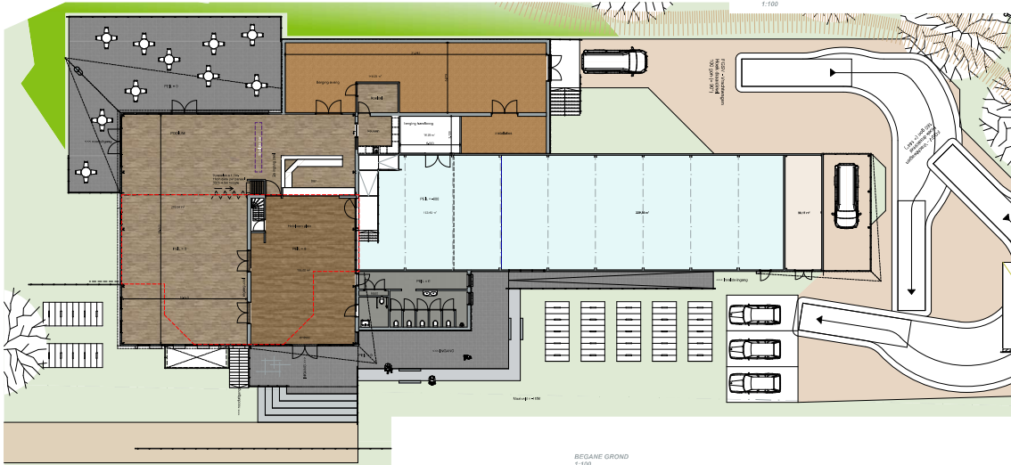
BEGANE GROND 1:100
