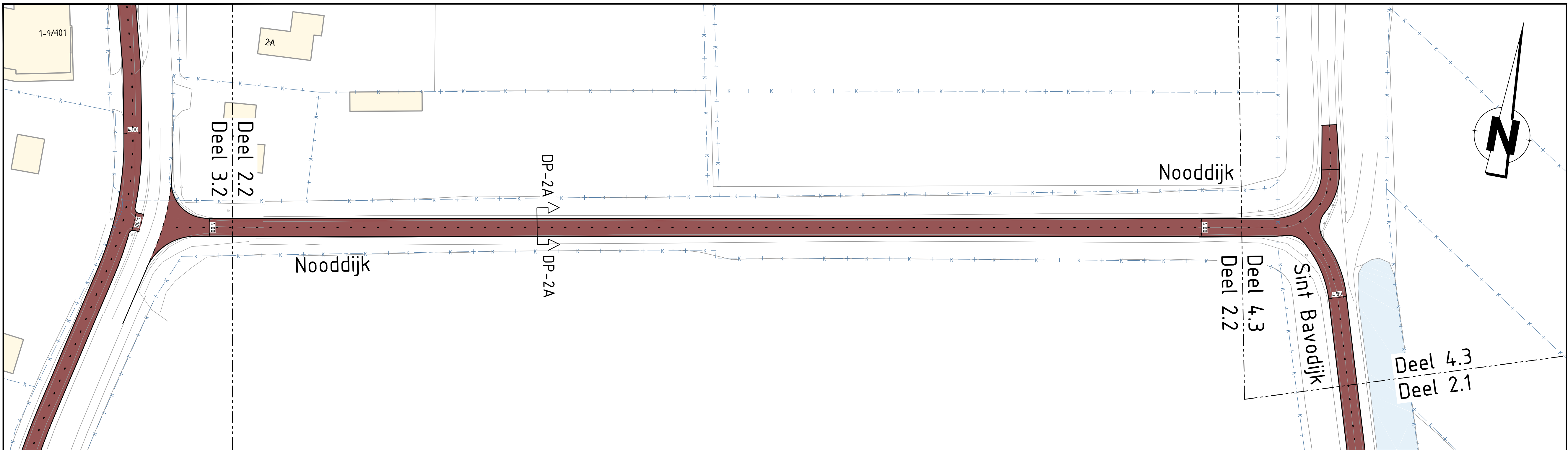
2.2 - Nieuwe situatie - B3 - Nooddijk SCHAAL 1 : 500
