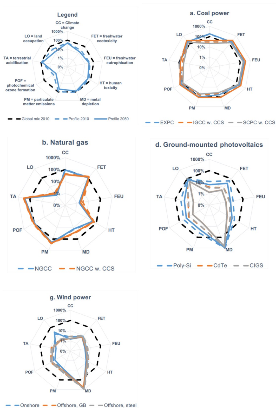
Afbeelding 5.27 Radardiagrammen met de impact op verschillende categorieën van kolen-, gas-, zon-, en windenergie relatief aan het wereldgemiddelde in 2010, aangegeven door de zwarte stippellijn. De verhouding is aangegeven op logaritmische schaal. Het gaat voor alle alternatieven in dit diagram om de blauwe stippellijn (EXPC bij kolen, NGCC bij gas, Poly-Si voor zon, en Onshore voor wind). Bron: (Gibon, Arvesen, & Hertwich, 2017)
