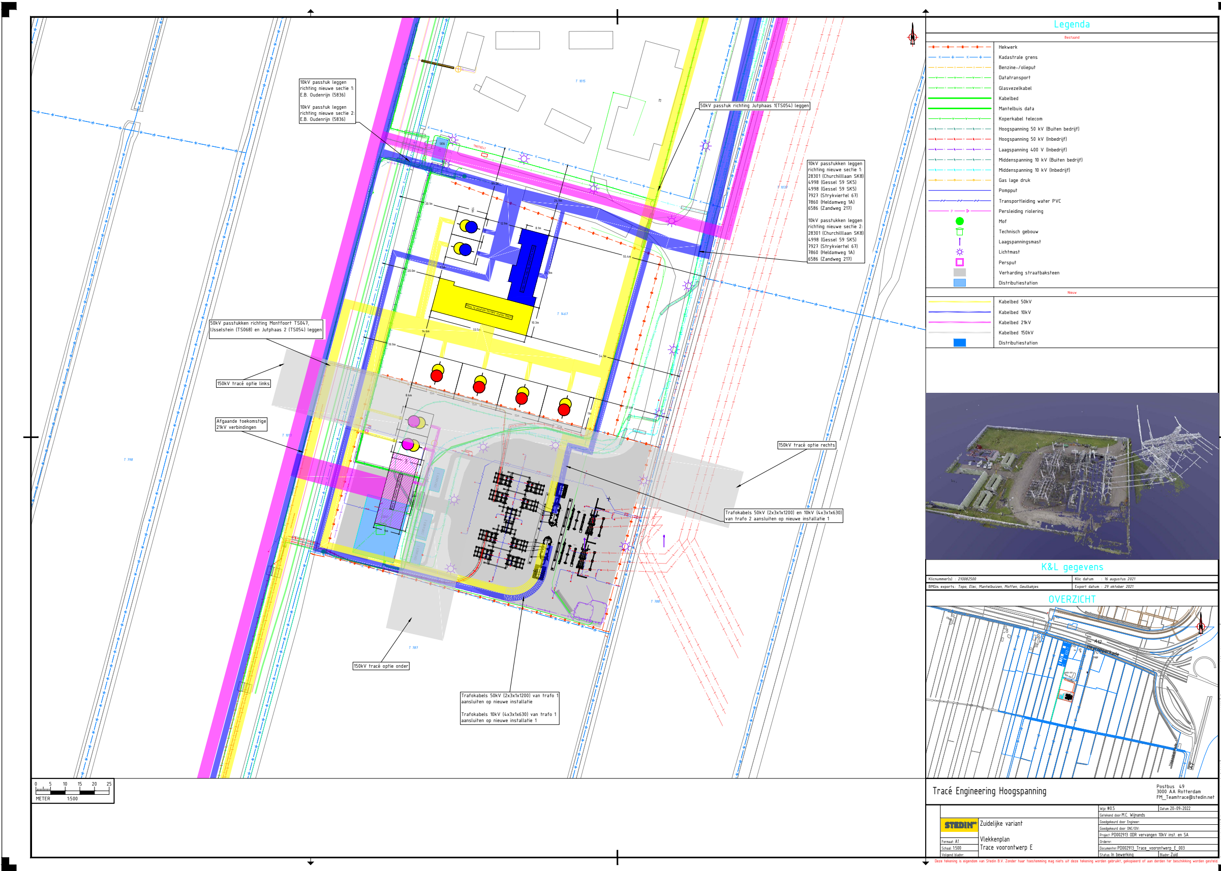
Landschappelijke inpassing 50kV en 10kV station Oudenrijn
