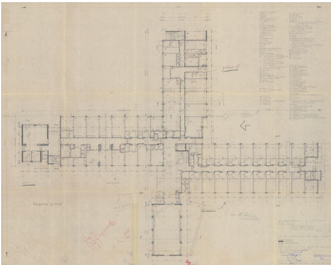
Ontwerp voor de begane grond, d.d. 24 juni 1969.
