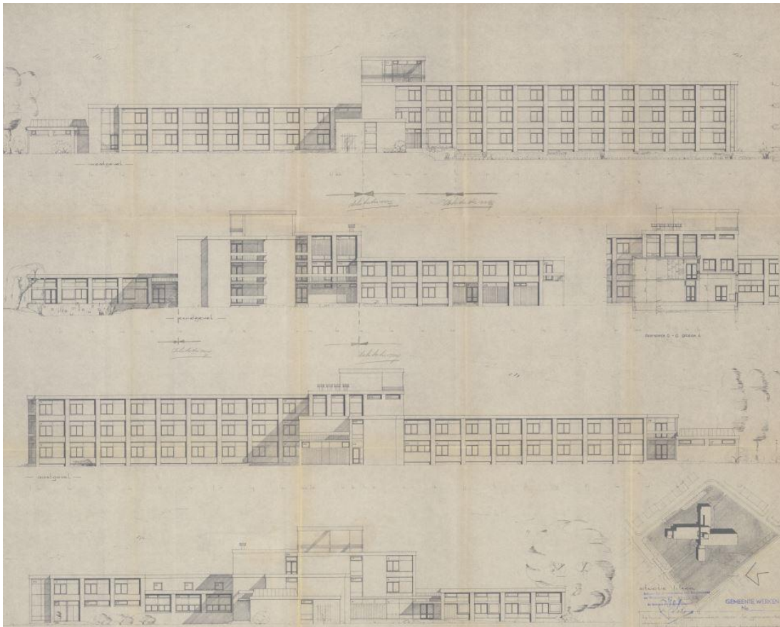
Gevelopstanden, d.d. 17 juni 1969.
